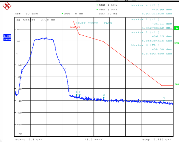
11N20MIMO Ant1 High 5825
