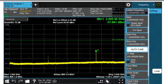
Band26(824-849)-3MHz-QPSK-26915-1RB#0-1000~3000-PASS
