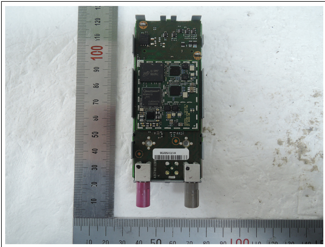
<LTE Module>
