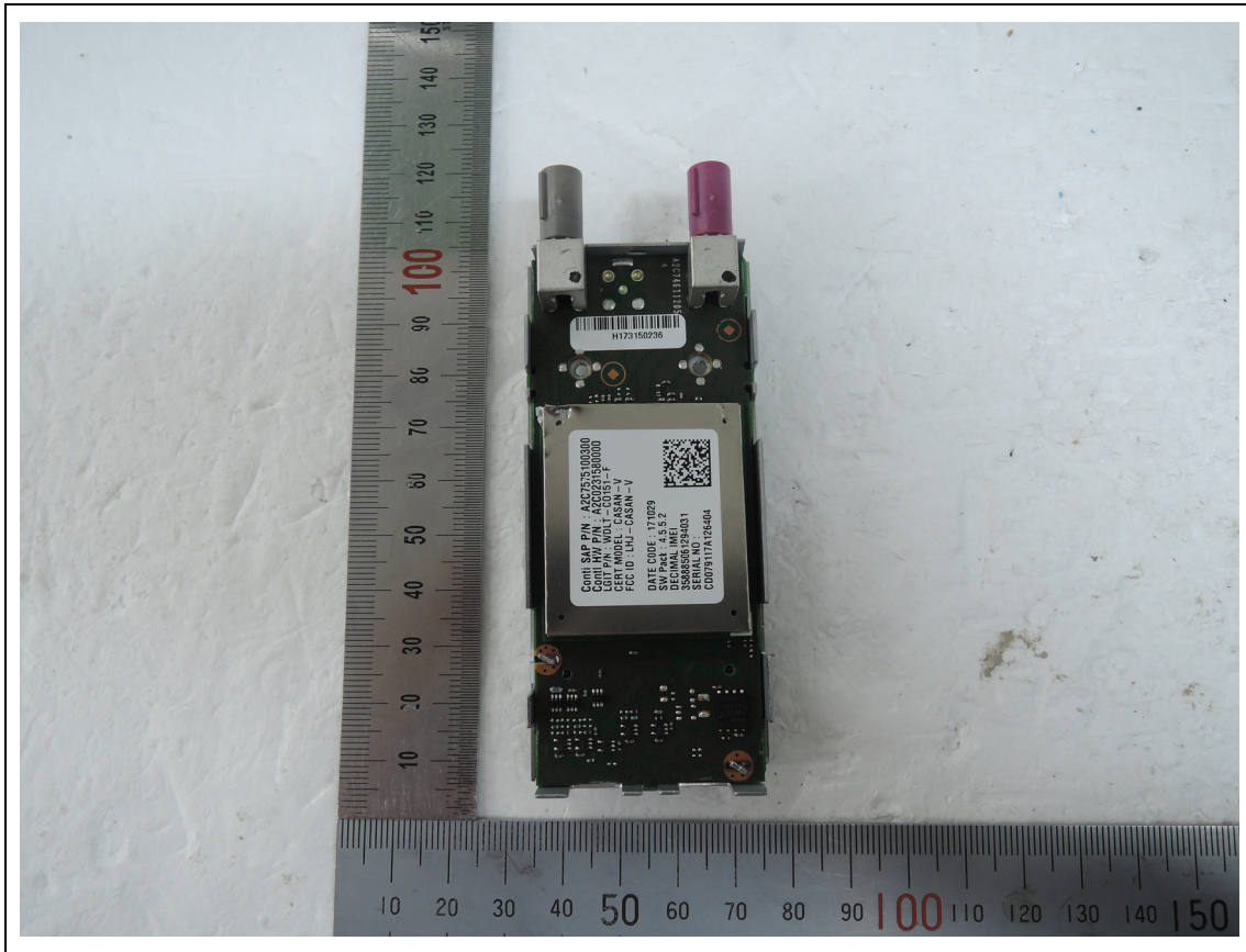
<LTE Module>
