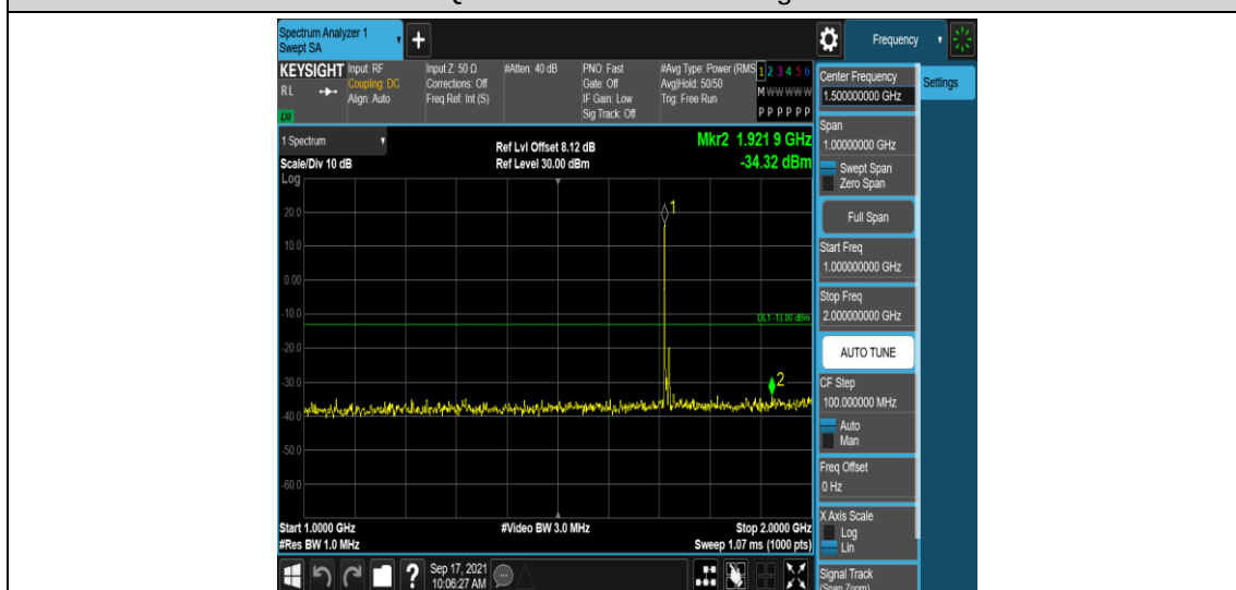
Band4-10MHz-QPSK-20000-1RB#0-Range4:1000~2000MHz
