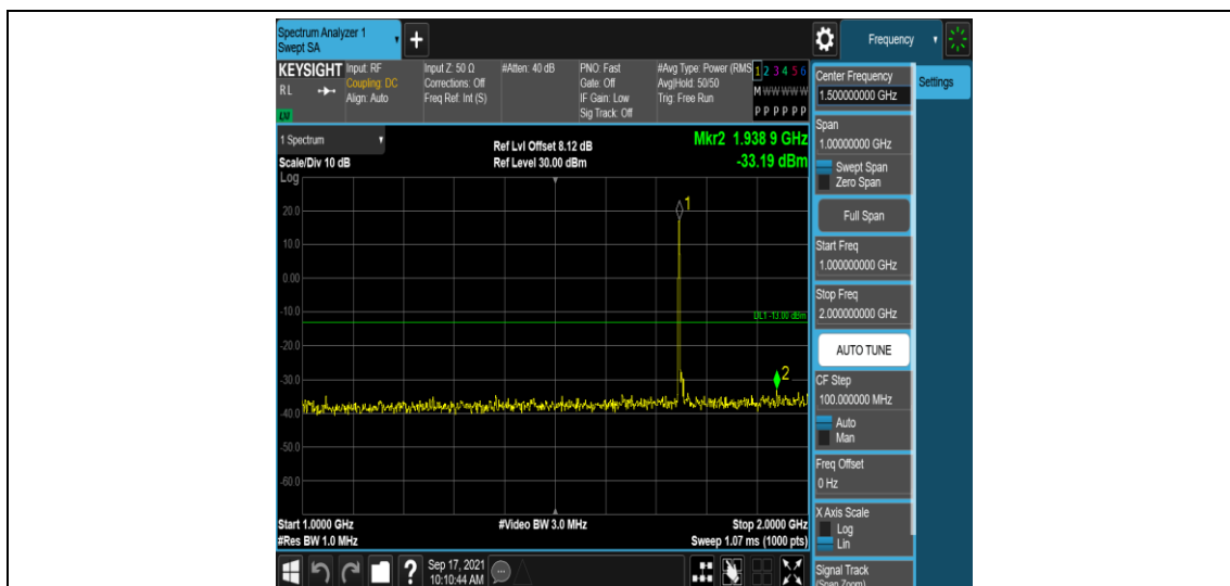
Band4-10MHz-QPSK-20350-1RB#0-Range4:1000~2000MHz
