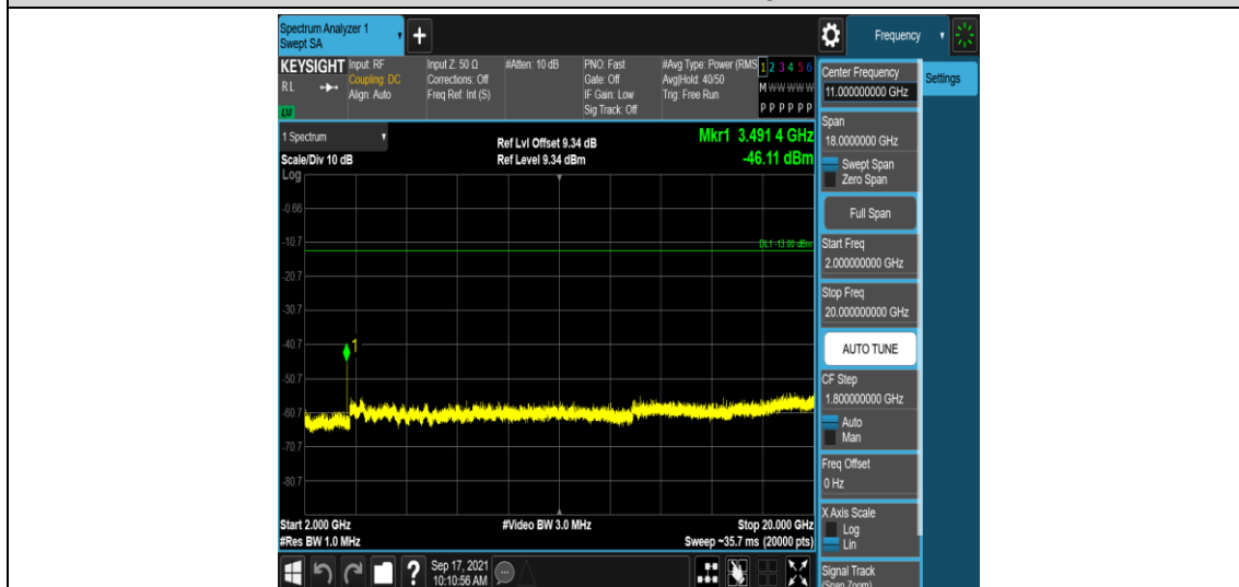
Band4-10MHz-QPSK-20350-1RB#0-Range5:2000~20000MHz
