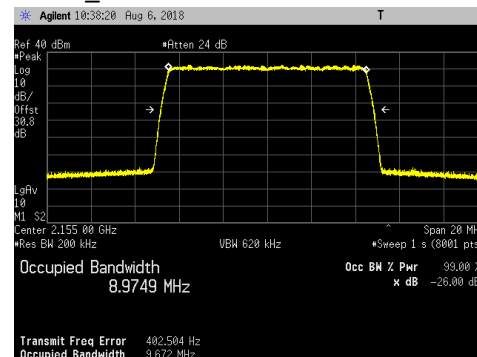
LTE10_64QAM
