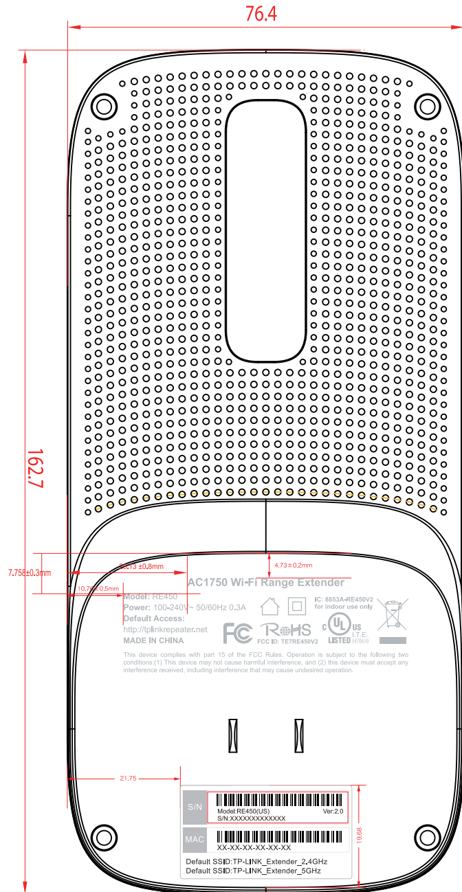
尺寸图
