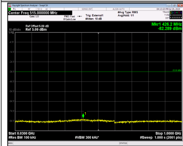
41-41-20MHz-10MHz-64QAM-64QAM-40571-40715-1RB #0-0RB#0-30~1000MHz-PASS
