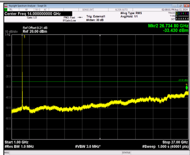
41-41-20MHz-5MHz-QPSK-QPSK-40595-40712-1RB#0-ORB#0- 1000~27000MHz-PASS
