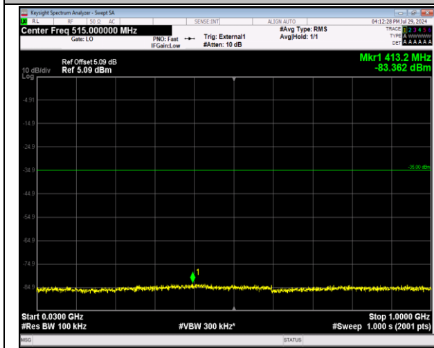
41-41-20MHz-10MHz-64QAM-64QAM-39750-39894-100 RB#0-50RB#0-30~1000MHz-PASS
