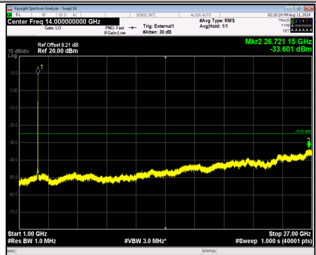
41-41-20MHz-5MHz-QPSK-QPSK-41440-41557-100RB#0-25RB#0-1000~27000MHz-PASS
