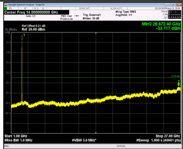
41-41-20MHz-5MHz-QPSK-QPSK-41440-41557-1RB#0-1RB#24-1000~27000MHz-PASS
