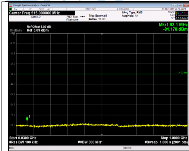
41-41-20MHz-10MHz-64QAM-64QAM-39750-39894-1RB #99-0RB#0-30~1000MHz-PASS
