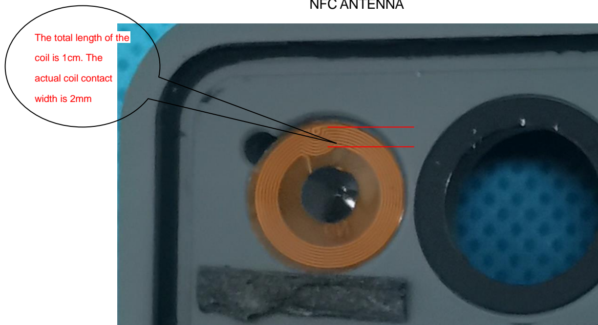
NFC ANTENNA
