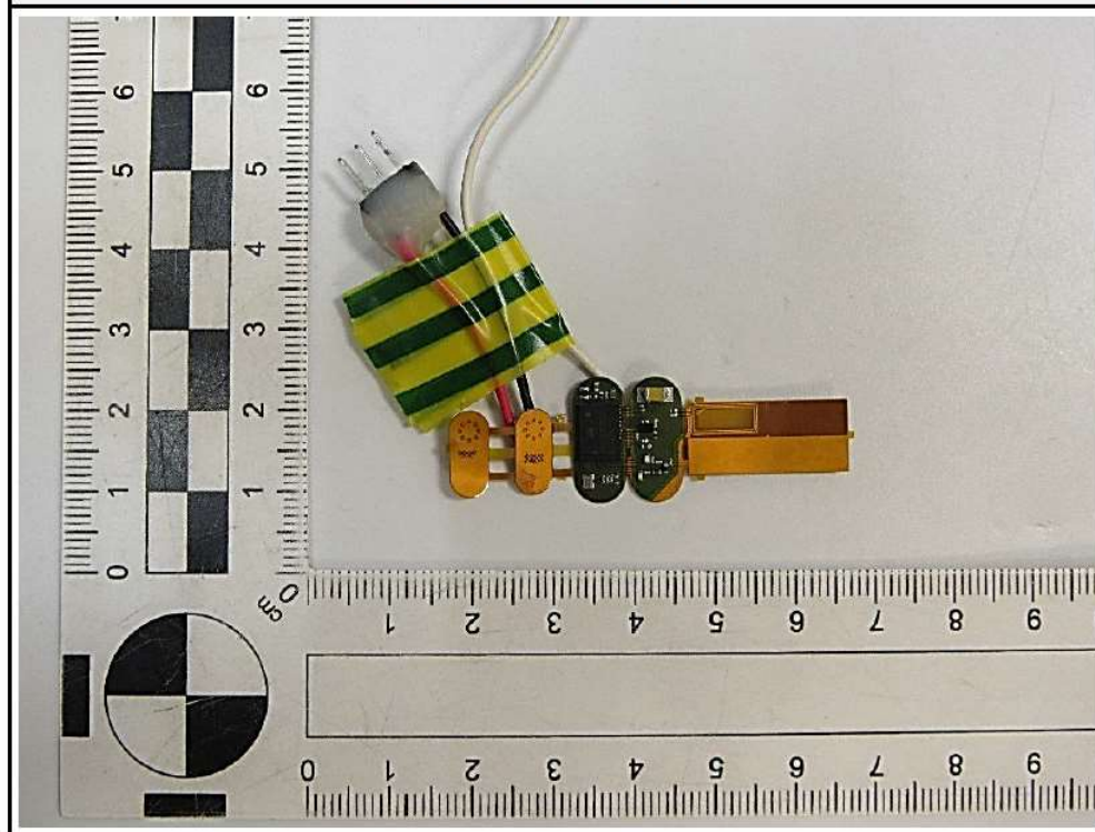
PCB top view - P024
