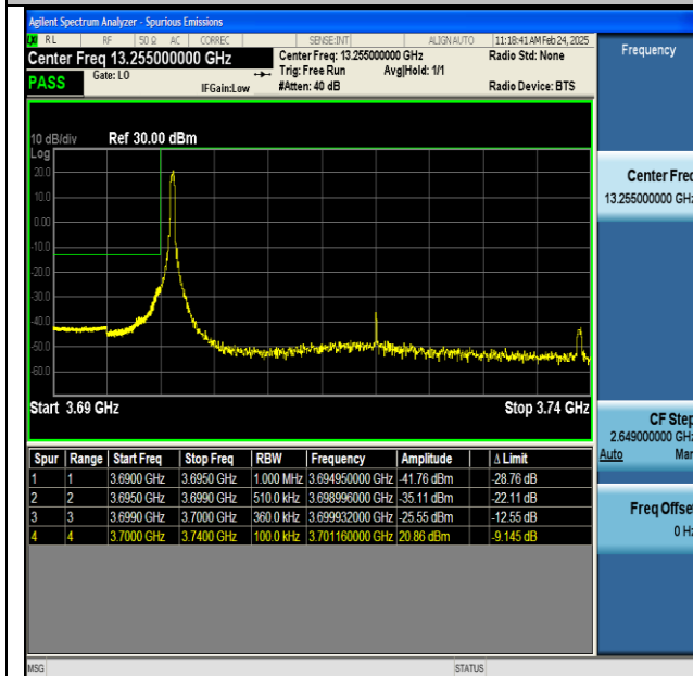
NTNV-n77(3700-3980)-PC2-30-40-L-CP-QPSK- Edge_1RB_Left-PASS
