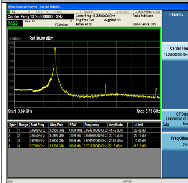
NTNV-n77(3700-3980)-PC2-30-30-L-CP-QPSK- Edge_1RB_Left-PASS
