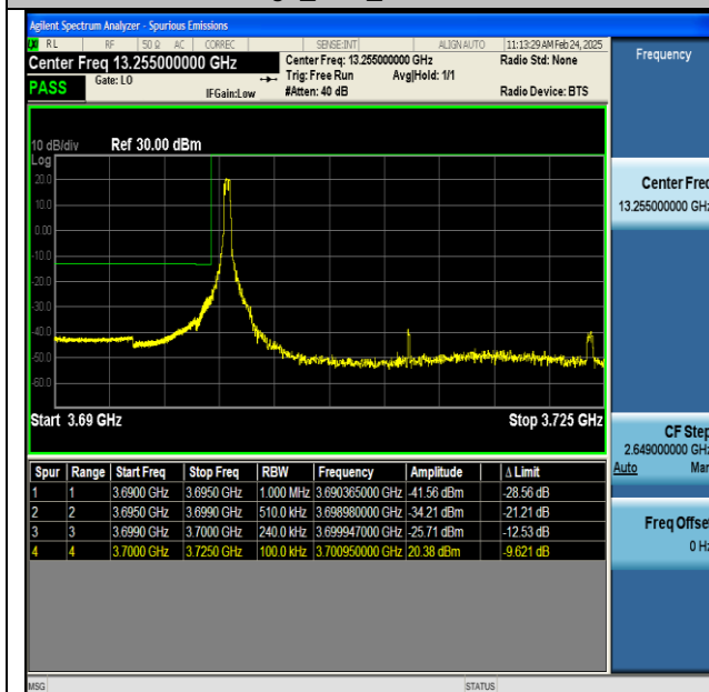
NTNV-n77(3700-3980)-PC2-30-25-L-CP-QPSK- Edge_1RB_Left-PASS
