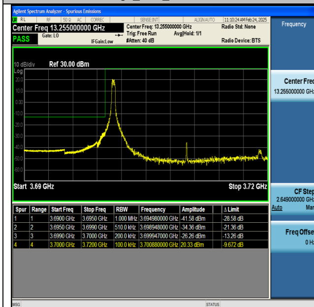
NTNV-n77(3700-3980)-PC2-30-20-L-CP-QPSK- Edge_1RB_Left-PASS
