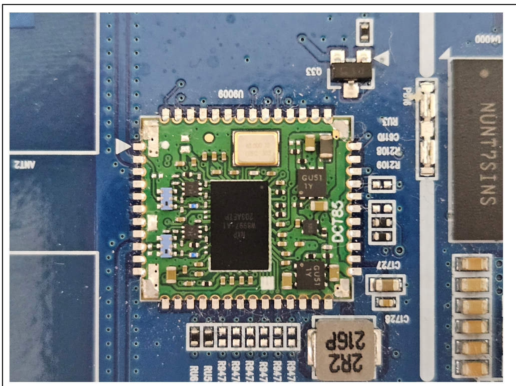
<WLAN Module>
