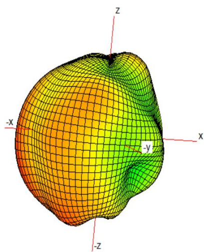
5500MHz
