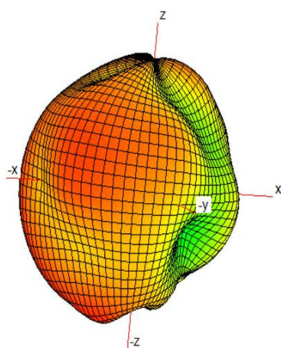
5800MHz
