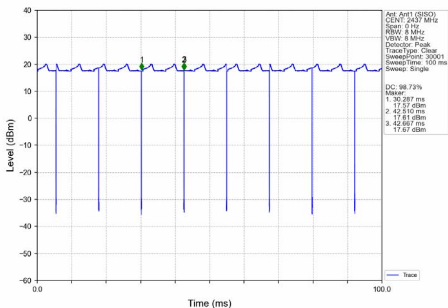
802.11b_MCH_2437MHz_Ant1 (SISO)_NTNV
