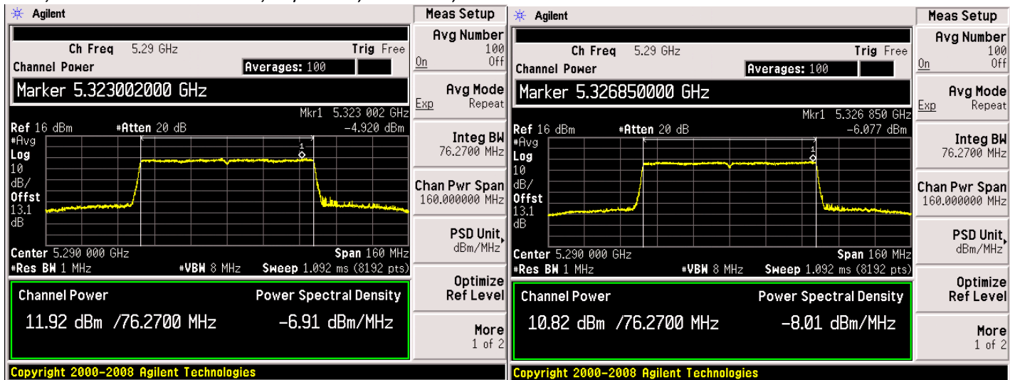
Antenna A
