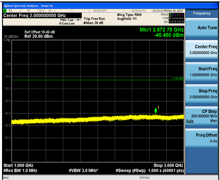
Band26 1.4MHz QPSK 27033 1RB#0 1000~3000 1000~3000
