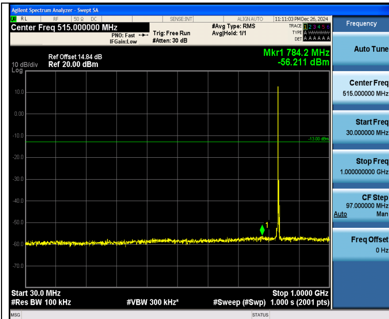
Band26 3MHz QPSK 26915 1RB#0 30~1000 30~1000
