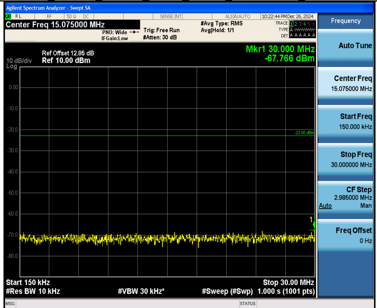
Band26 1.4MHz_QPSK 27033 1RB#0 0.15~30 0.15~30
