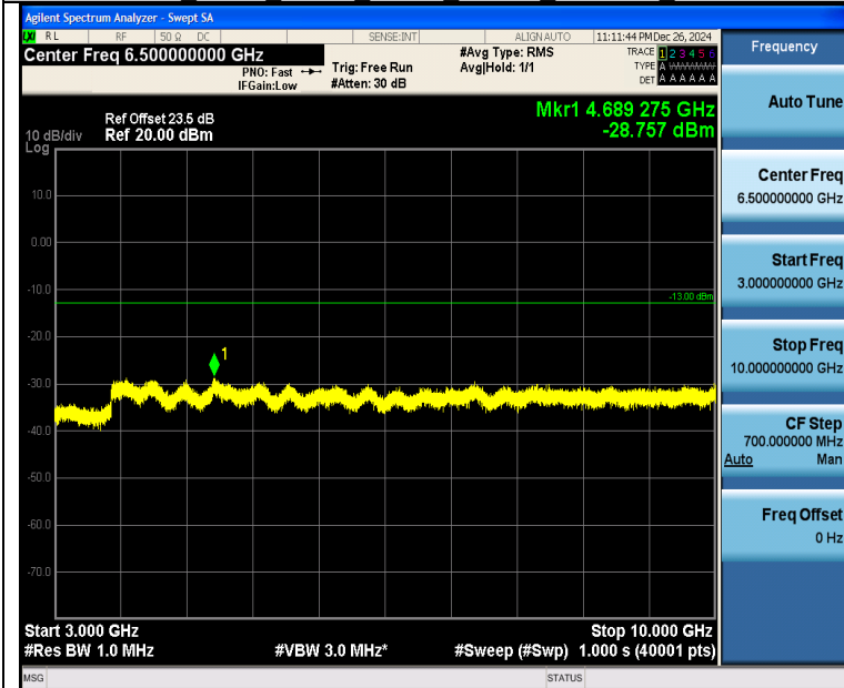
Band26 3MHz QPSK 26915 1RB#0 3000~10000 3000~10000
