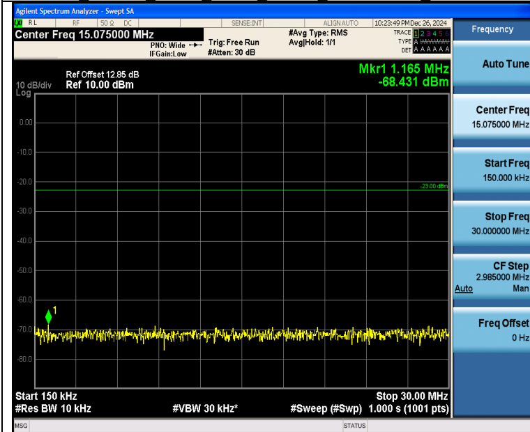
Band26 1.4MHz 16QAM 27033 1RB#0 0.15~30 0.15~30
