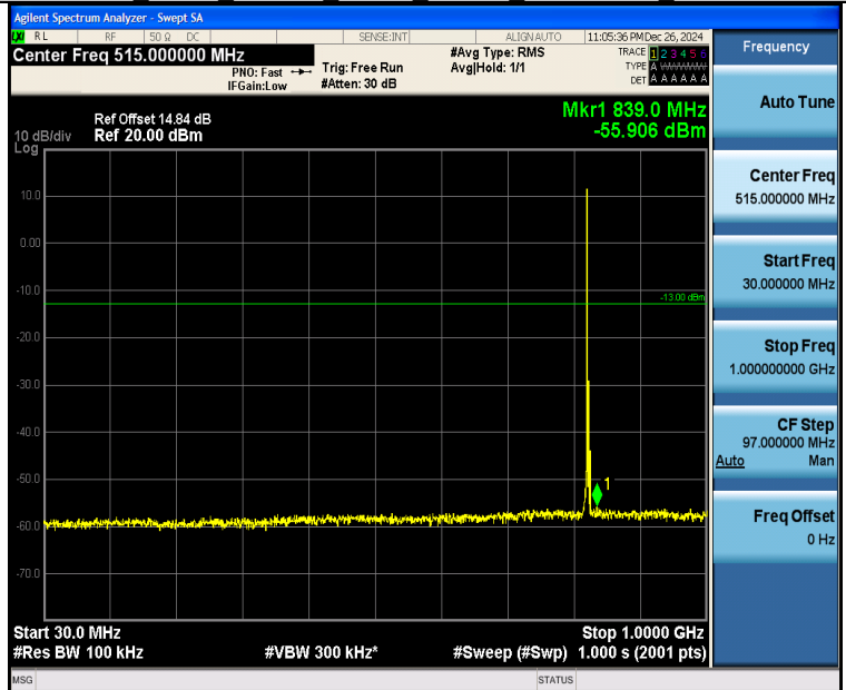
Band26 3MHz 16QAM 26805 1RB#0 30~1000 30~1000
