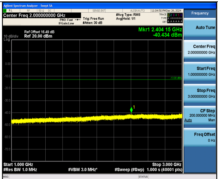
Band26 3MHz QPSK 26805 1RB#0 1000~3000 1000~3000
