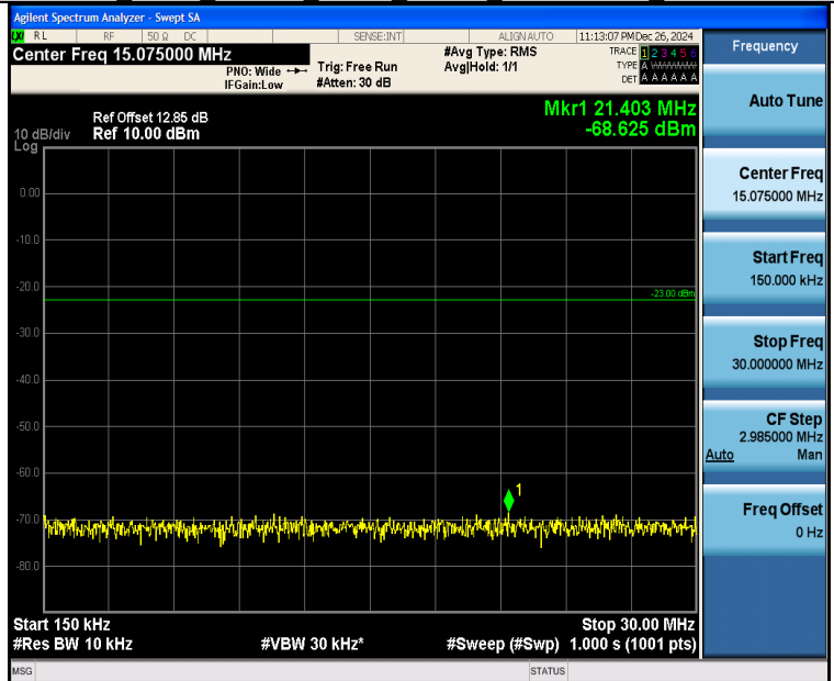
Band26 3MHz QPSK 26915 1RB#14 0.15~30 0.15~30
