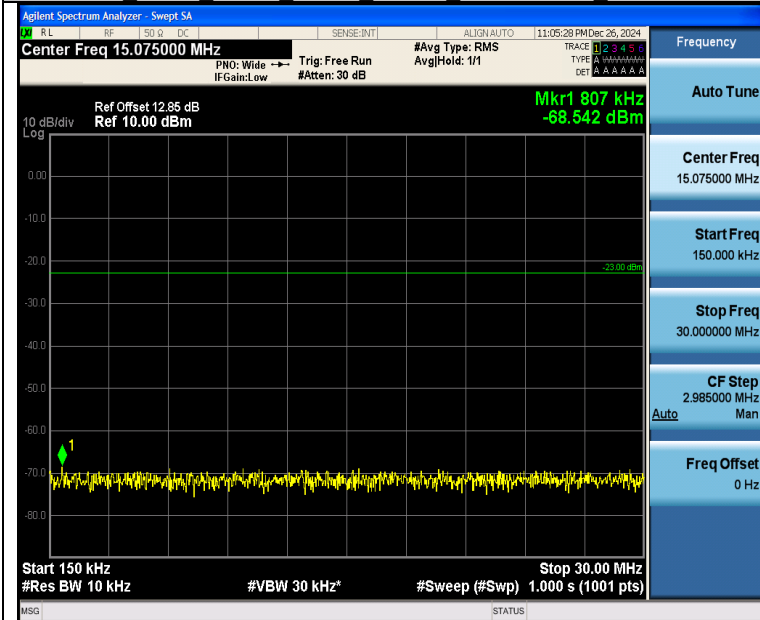
Band26 3MHz 16QAM 26805 1RB#0 0.15~30 0.15~30
