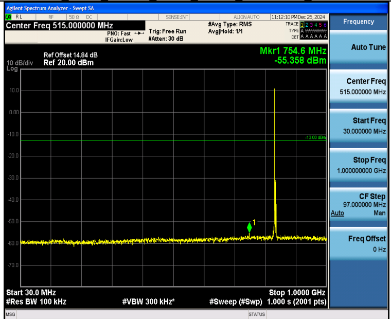
Band26 3MHz 16QAM 26915 1RB#0 30~1000 30~1000
