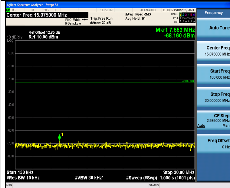
Band26 3MHz 16QAM 27025 1RB#0 0.15~30 0.15~30
