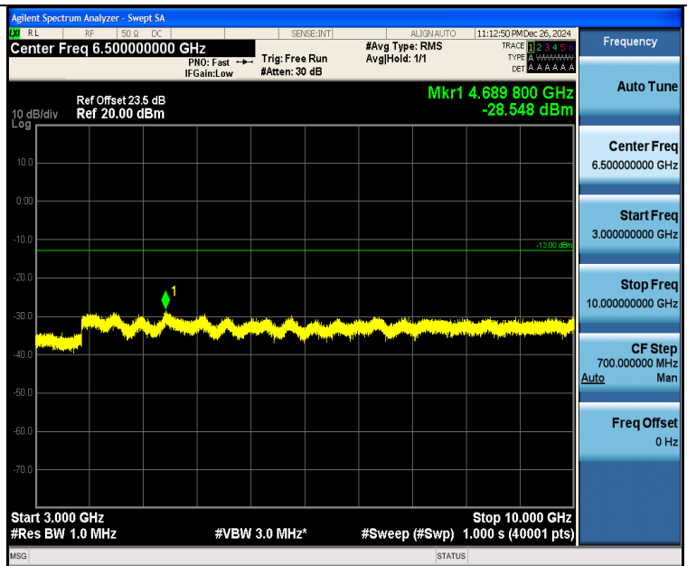
Band26 3MHz 16QAM 26915 1RB#0 3000~10000 3000~10000
