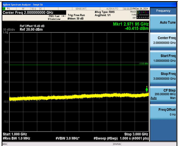
Band26 3MHz QPSK 26915 1RB#0 1000~3000 1000~3000
