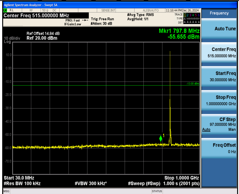
Band26 3MHz 16QAM 27025 1RB#0 30~1000 30~1000
