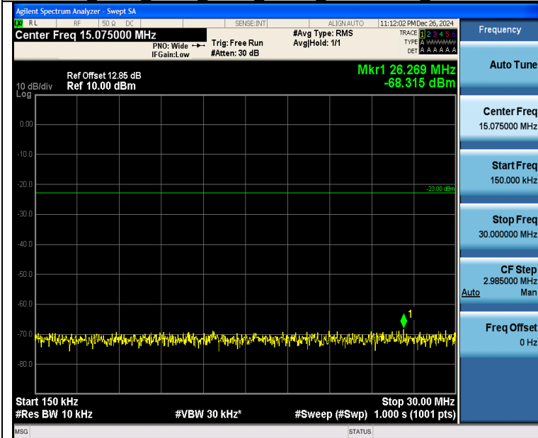
Band26 3MHz 16QAM 26915 1RB#0 0.15~30 0.15~30
