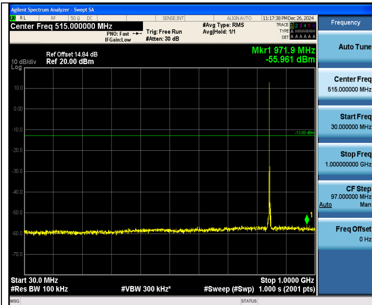
Band26 3MHz QPSK 27025 1RB#0 30~1000 30~1000
