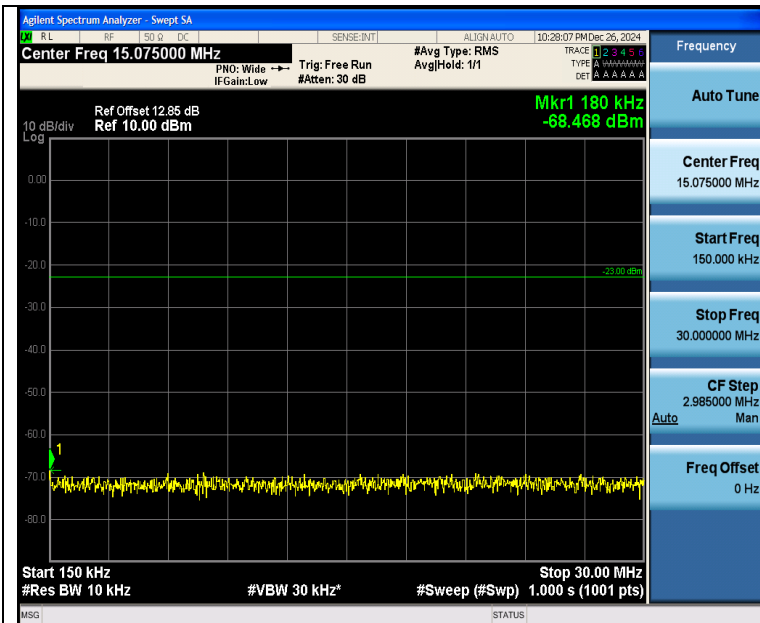
Band26 1.4MHz 16QAM 27033 6RB#0 0.15~30 0.15~30
