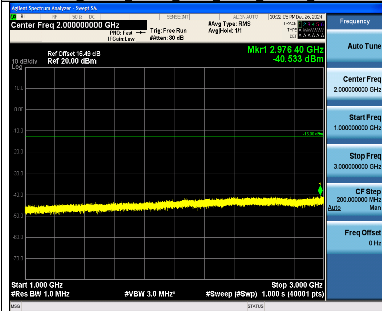
Band26 1.4MHz 16QAM 26915 6RB#0 1000~3000 1000~3000
