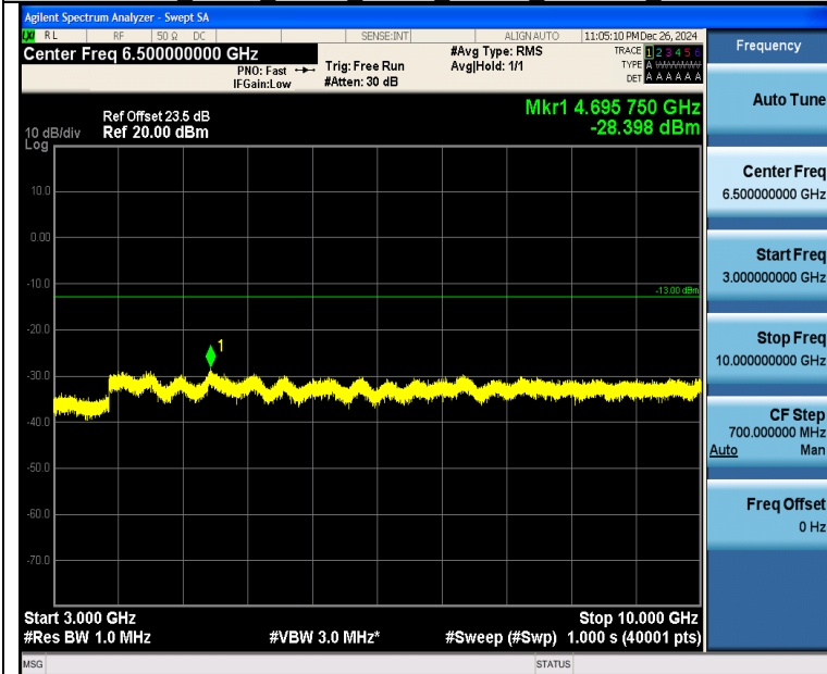
Band26 3MHz QPSK 26805 1RB#0 3000~10000 3000~10000
