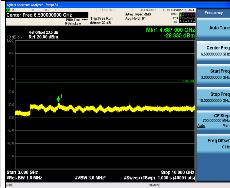
Band26 3MHz QPSK 27025 1RB#0 3000~10000 3000~10000
