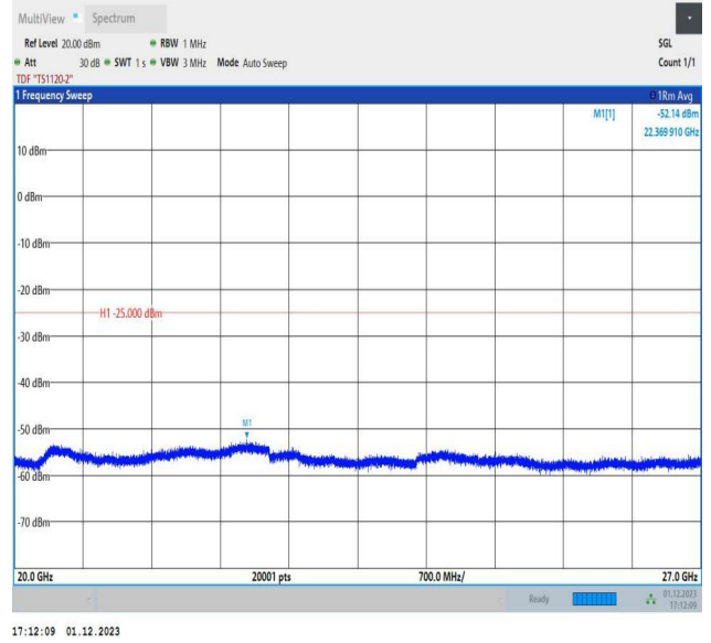
7-7-15MHz-20MHz-QPSK-QPSK-20828-20999-75RB#0-100R B#0-20000~27000MHz-PASS
