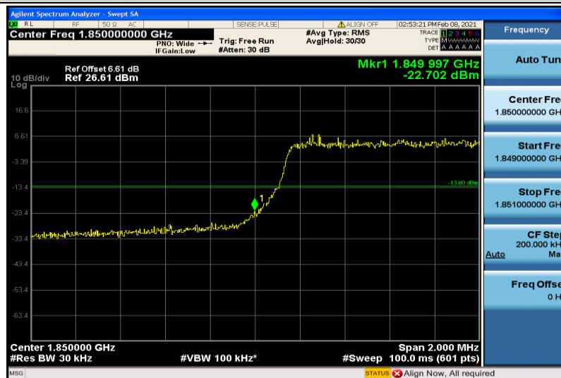
Band2-3MHz-QPSK-18615-6RB#0
