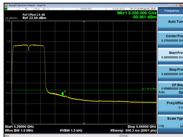
5310MHz AV
