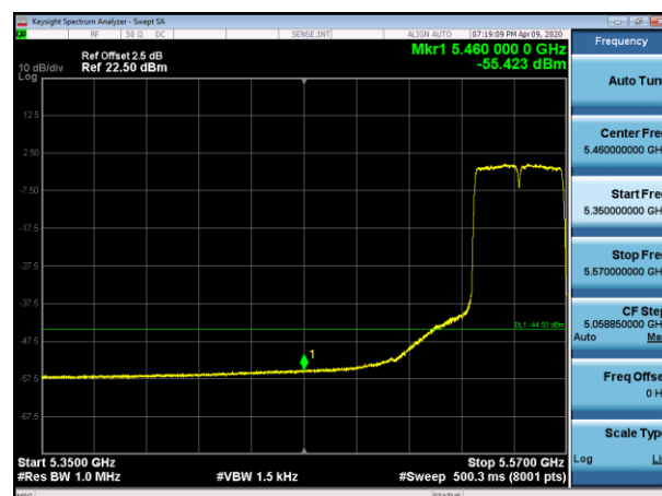
5550MHz AV
