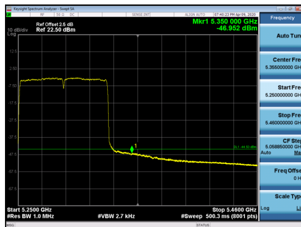
5290MHz AV
