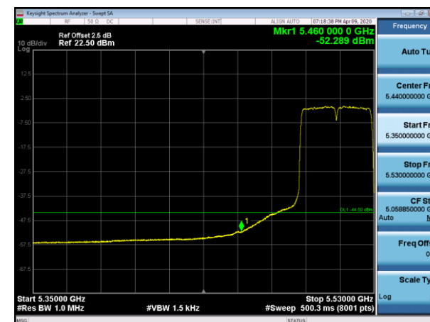
5510MHz AV
