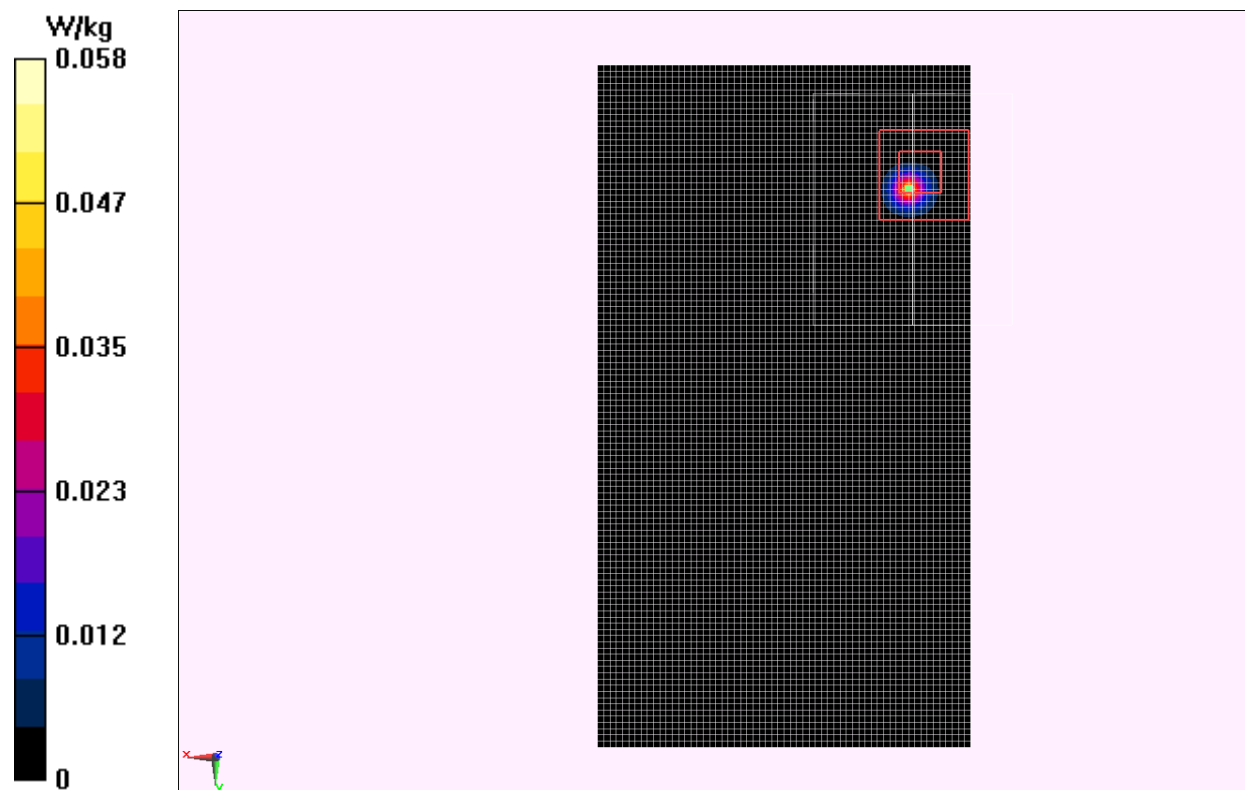
Fig.12 5GHz CH112
