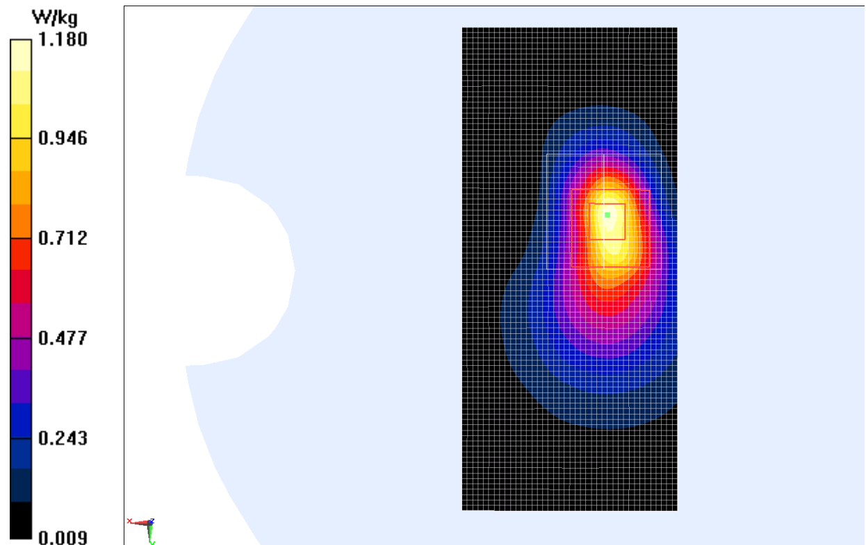
Fig.8 WCDMA1900 CH9538
