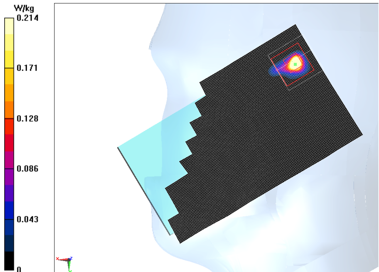
Fig.11 5GHz CH56
