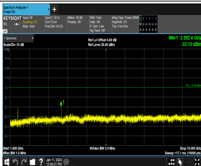
Band71-5MHz-QPSK-133297-1RB#0-Range2:1000~10000MHz
