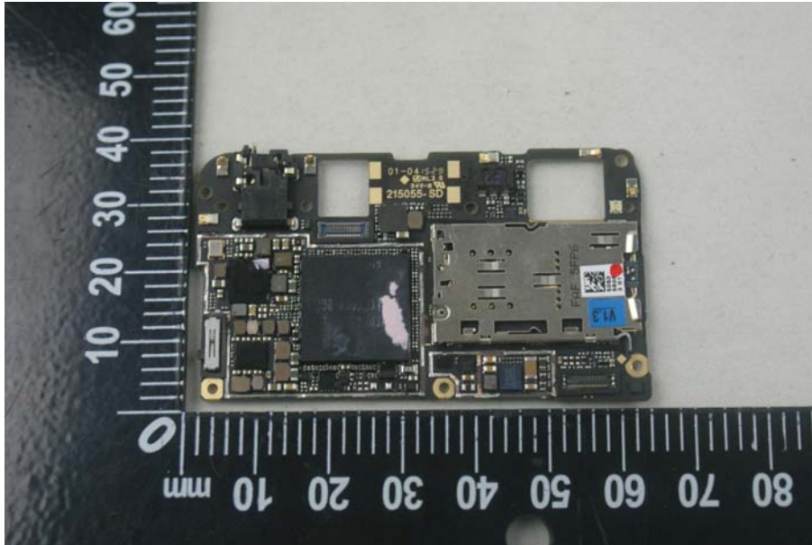
EUT Photo 7
