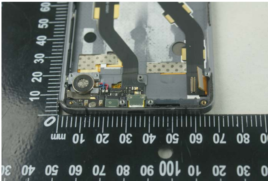
EUT Photo 8
