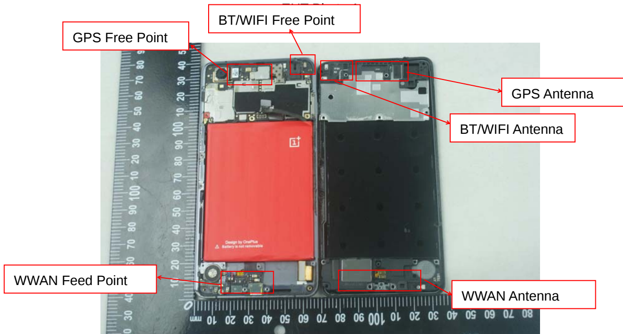
EUT Photo 2
