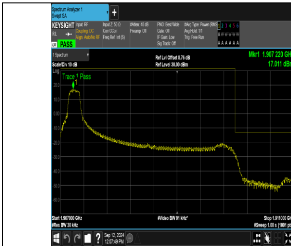
Band2_3MHz_QPSK_19185_1RB#0
