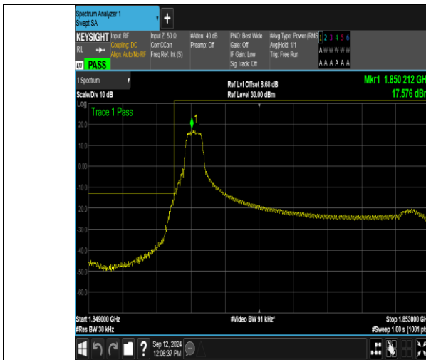
Band2_3MHz_QPSK_18615_1RB#0
