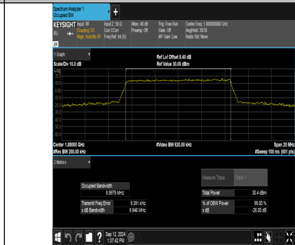
Band2-10MHz-16QAM-18900-50RB#0-PASS
