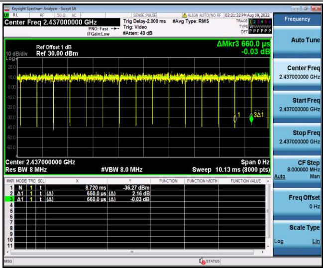
11N40SISO_Ant2_2437
