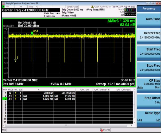
11N20SISO_Ant2_2412
