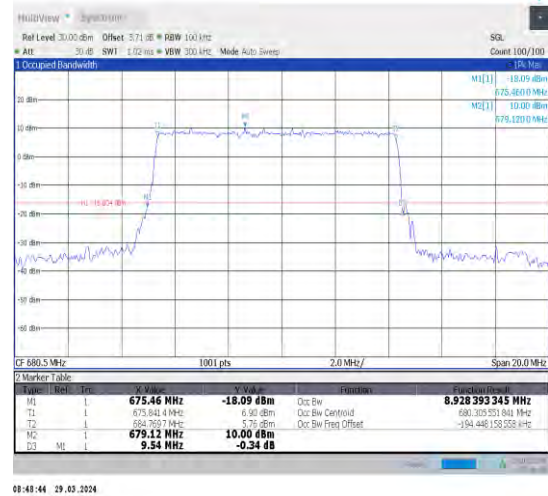
1-N71-15-10-M-5-DFT-256QAM-Outer_Full-50@0-A nt1-8.928-9.540-≤10-PASS
