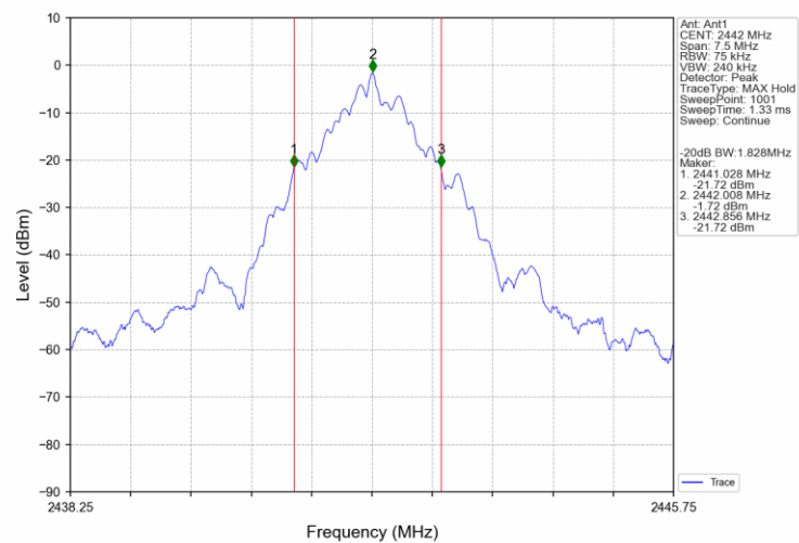
1_MCH_2442MHz_Ant1_NTNV
