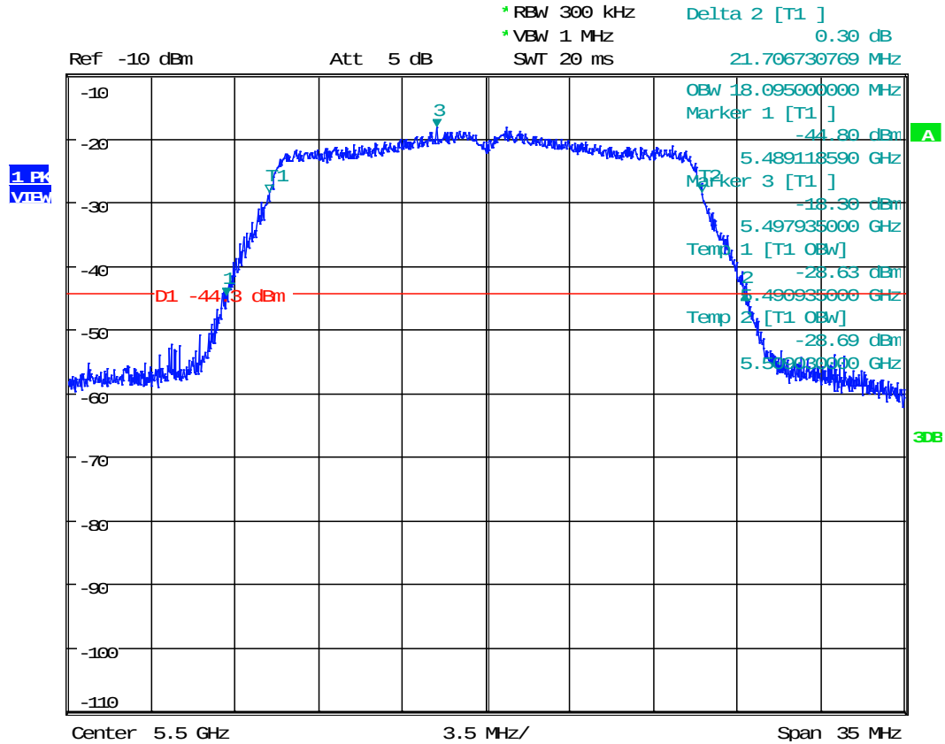
Plot 1. 4 802.11n 20MHz, 5500MHz
