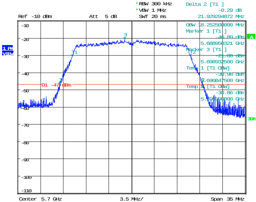
Plot 1. 6 802.11n 20MHz, 5700MHz
