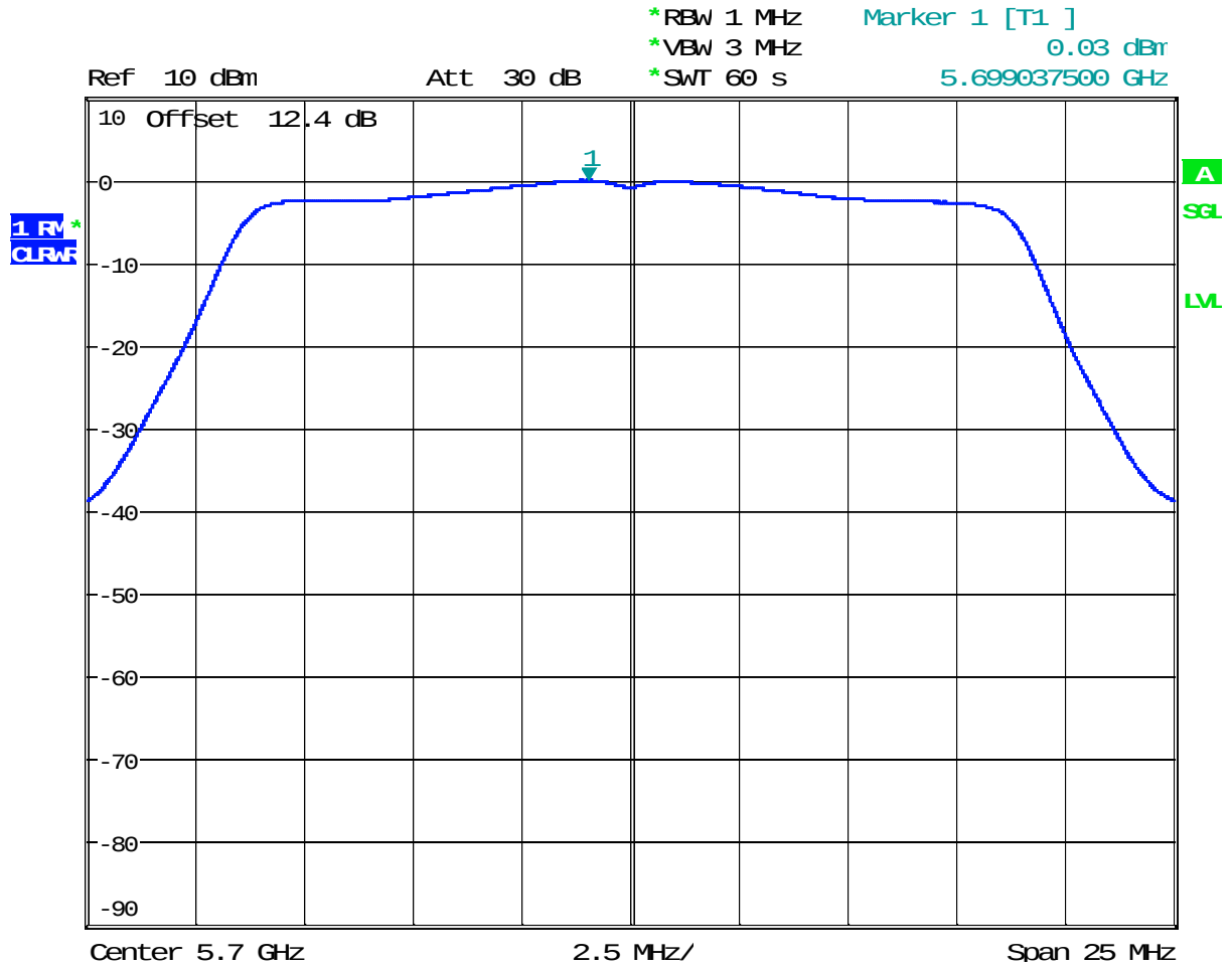
Plot 3. 14 802.11n 20MHz, 5700MHz
