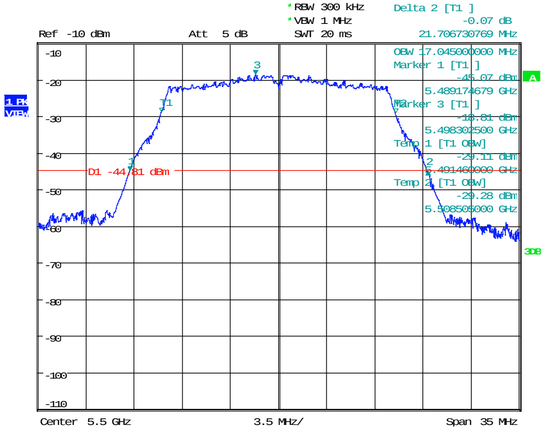
Plot 1. 1 802.11a 5500MHz
