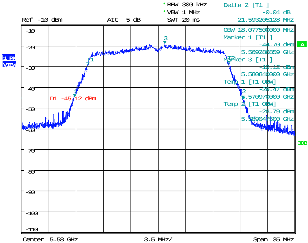
Plot 1.5 802.11n 20MHz, 5580MHz
