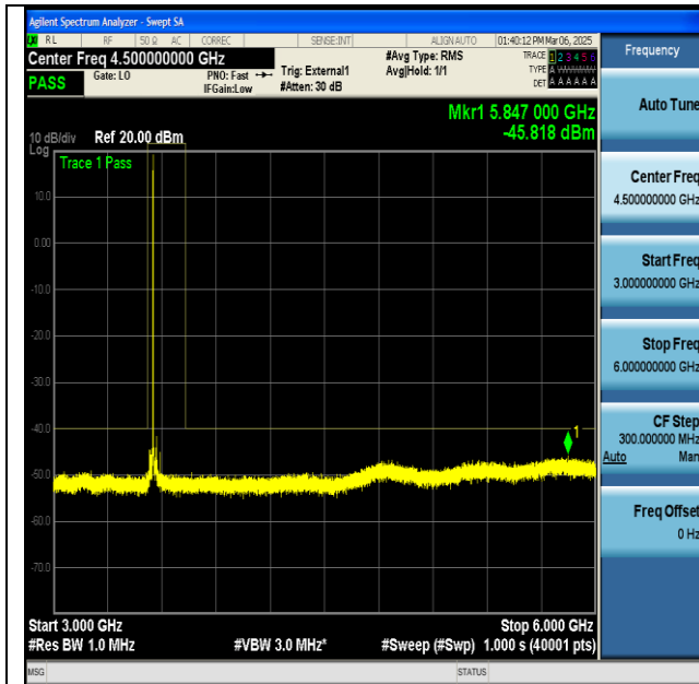
NTNV-n48-PC3-30-40-L-CP-QPSK-Edge_1RB_Left-3000-6000-PASS
