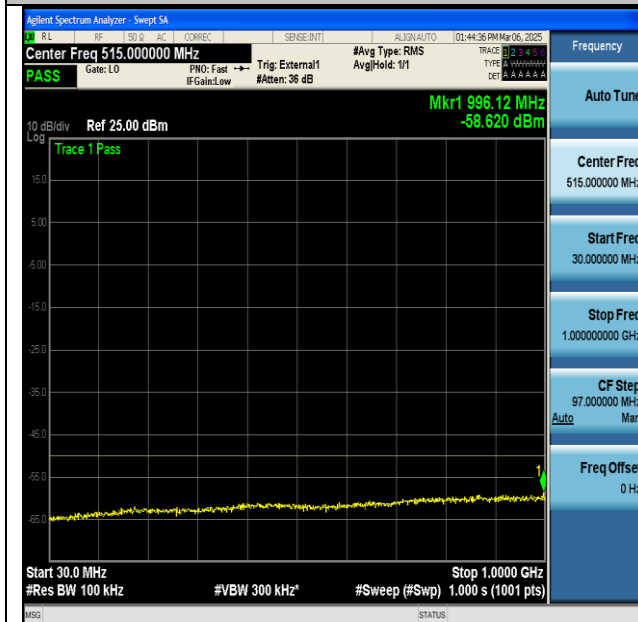
NTNV-n48-PC3-30-40-M-CP-QPSK-Edge_1RB_Left-30- 1000-PASS
