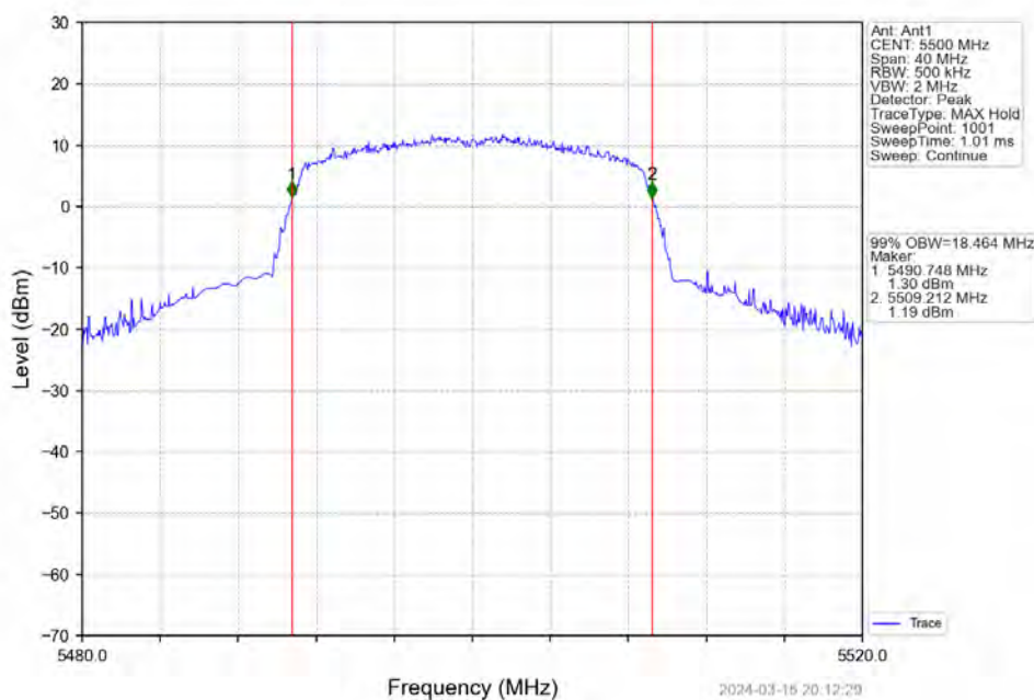
802.11n(HT20)_LCH_5500MHz_Ant7_NTNV
