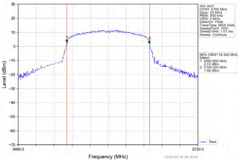
802.11n(HT20)_HCH_5700MHz_Ant7_NTNV
