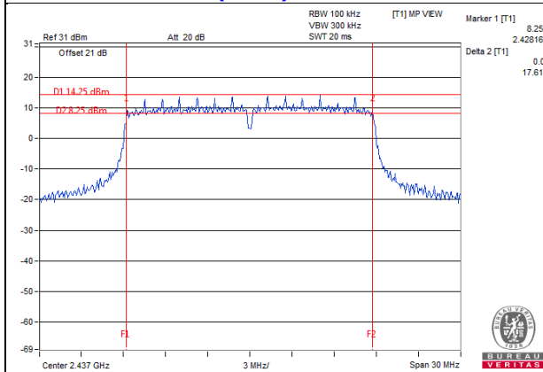
802.11n (HT20)_Chain 0 / CH6
