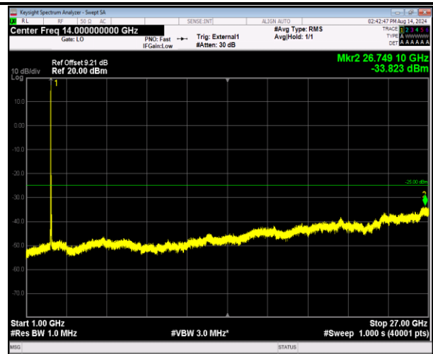
41-41-20MHz-20MHz-QPSK-QPSK-40641-40839-1RB#0-0 RB#0-1000~27000MHz-PASS
