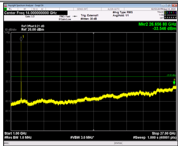
41-41-20MHz-20MHz-QPSK-QPSK-40942-41140-1RB#0-1 RB#99-1000~27000MHz-PASS
