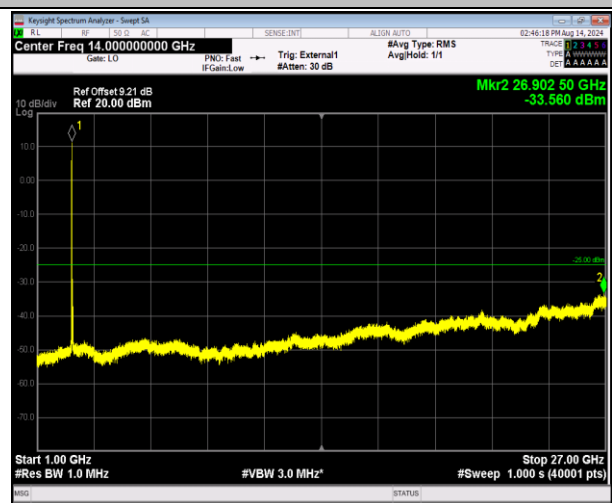
41-41-20MHz-20MHz-QPSK-QPSK-40641-40839-1RB#0-1 RB#99-1000~27000MHz-PASS
