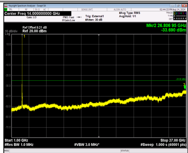
41-41-20MHz-20MHz-QPSK-QPSK-40641-40839-1RB#99- ORB#0-1000~27000MHz-PASS
