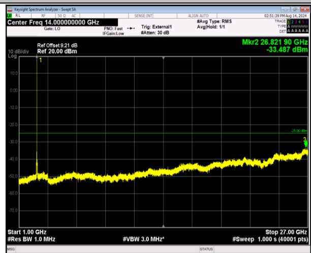
41-41-20MHz-20MHz-QPSK-QPSK-40942-41140-1RB#99- ORB#0-1000~27000MHz-PASS
