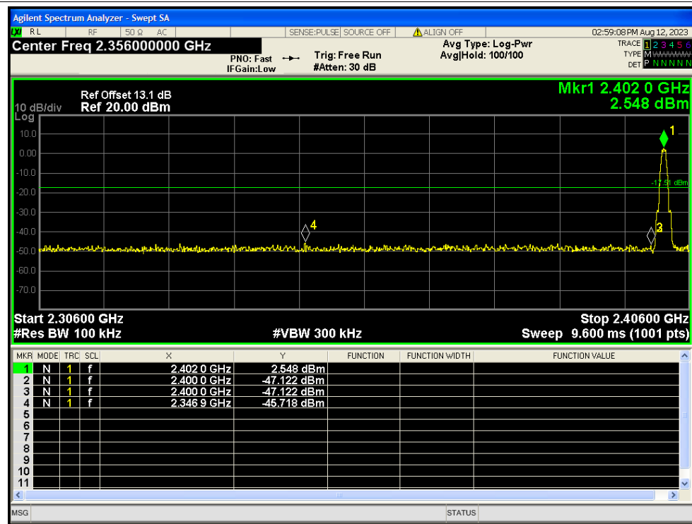
Band Edge NVNT BLE 1M 2402MHz Ant1 Emission SISO
