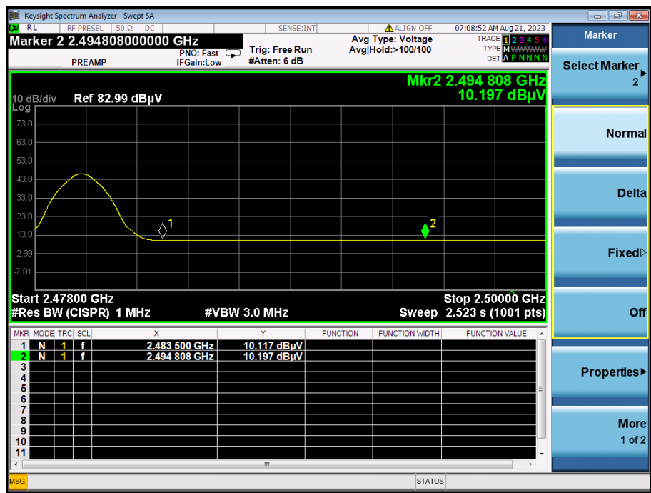
(AVERAGE, Channel 39)
