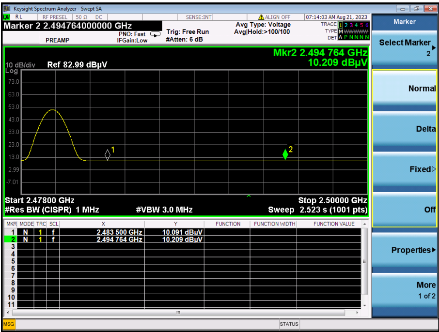
(AVERAGE, Channel 39)
