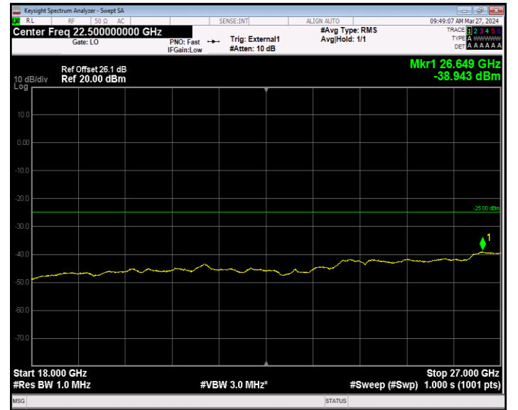
Band41_5MHz_16QAM_39675_1RB#0_18000~27000_18000~27000 000
