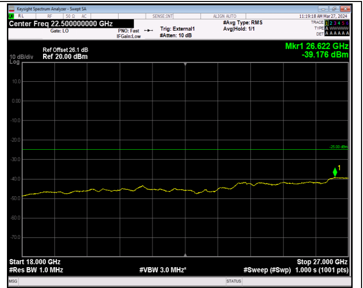
Band41_20MHz_QPSK_39750_1RB#0_18000~27000_18000~27 000
