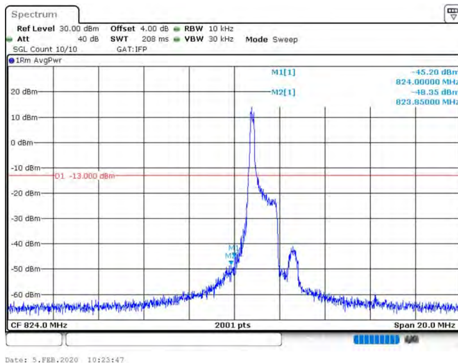
B26_CH26840_10M_QPSK_1RB0 (Part 22)
