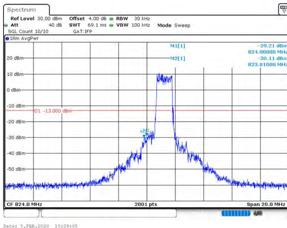
B26_CH26840_10M_QPSK_6RB0 (Part 22)
