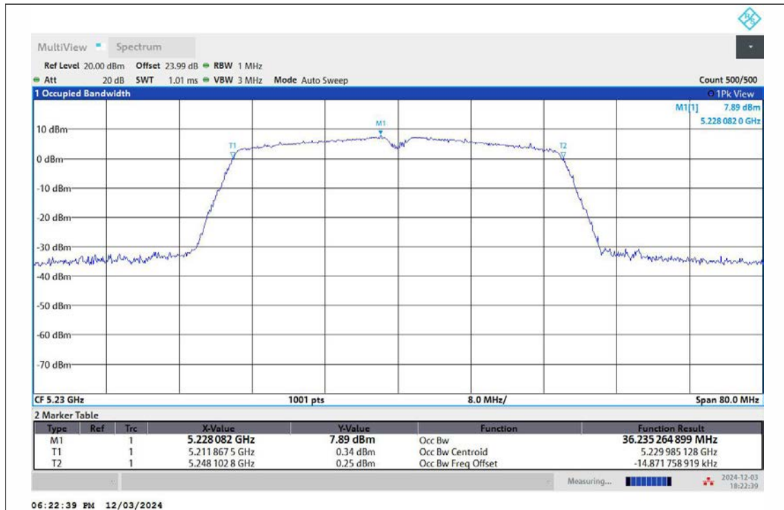
11AC40MIMO-Ant1-5230
