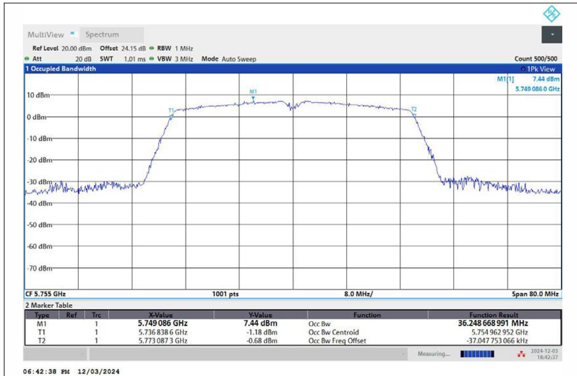
11AC40MIMO-Ant1-5755
