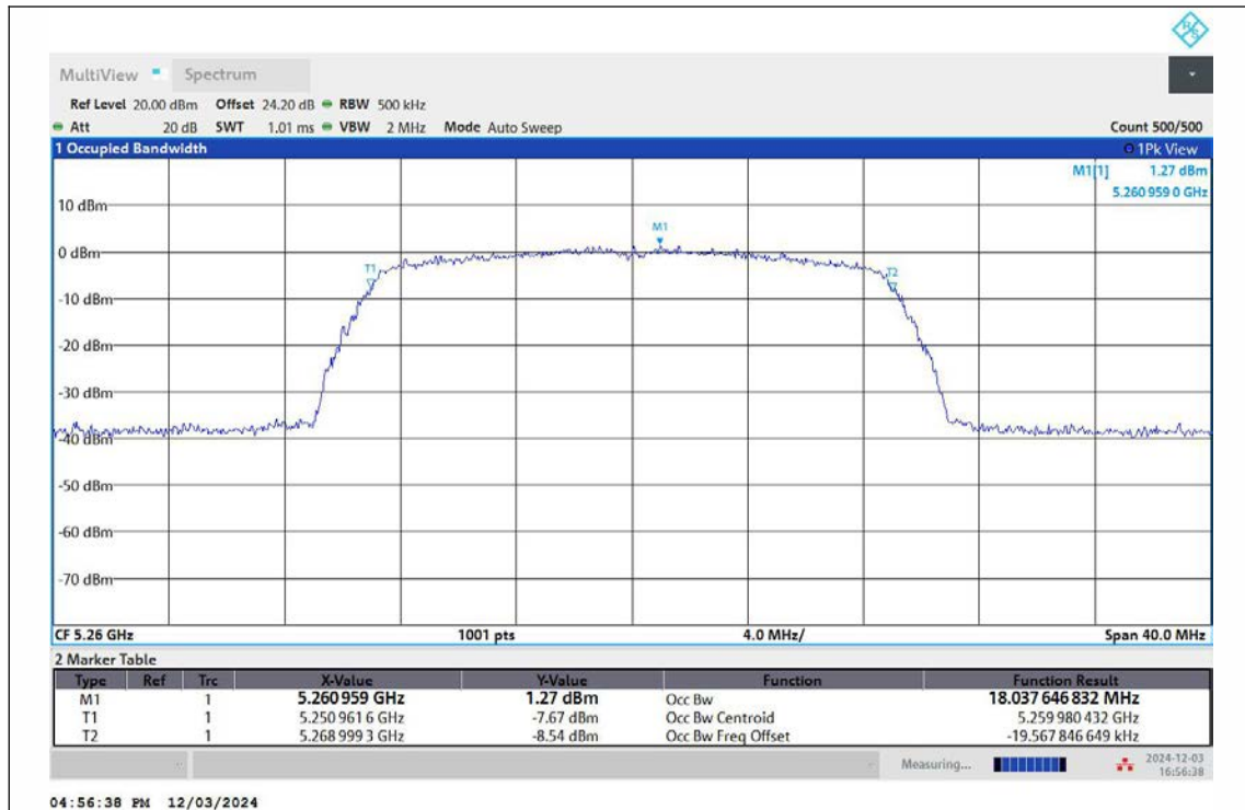
11AC20MIMO-Ant1-5260
