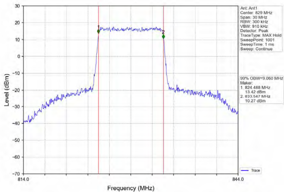
Band5_10MHz_QPSK_LCH_829MHz_RB_50_0_NTNV
