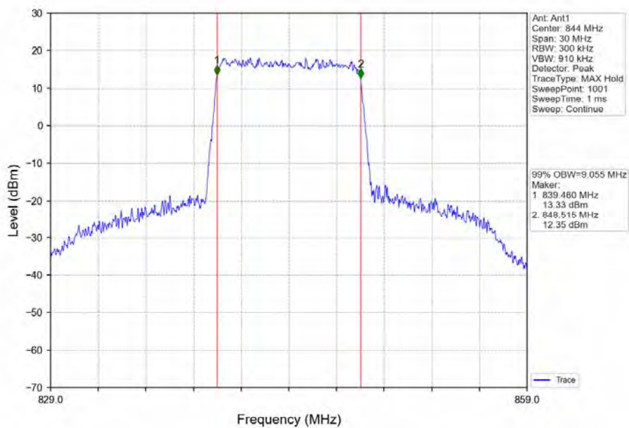
Band5_10MHz_QPSK_HCH_844MHz_RB_50_0_NTNV
