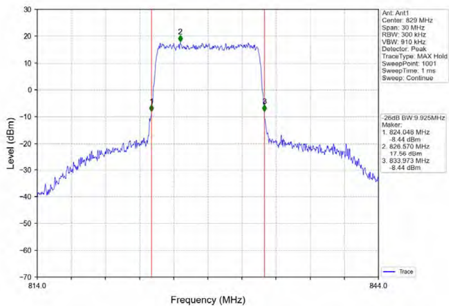
Band5_10MHz_QPSK_LCH_829MHz_RB_50_0_NTNV
