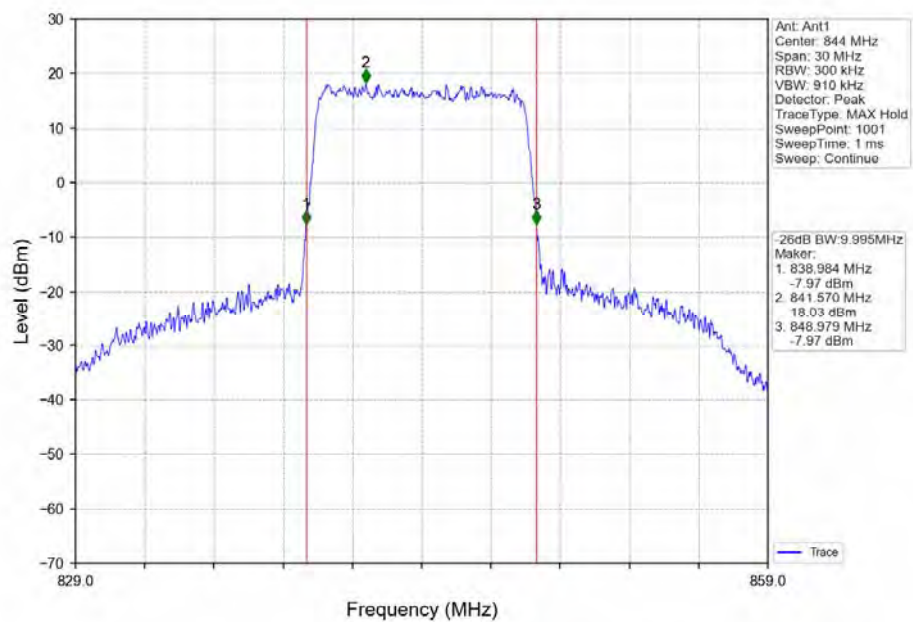
Band5_10MHz_QPSK_HCH_844MHz_RB_50_0_NTNV
