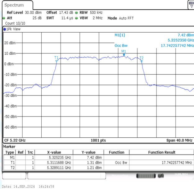
11N20MIMO-Ant1-5320
