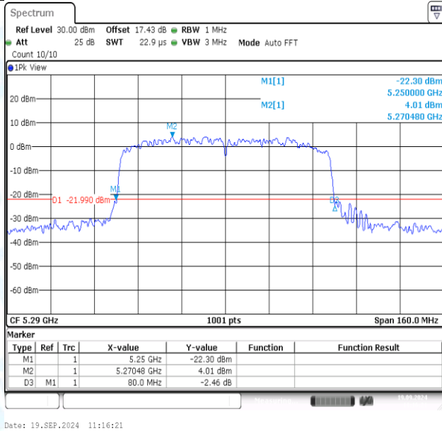
11AC80MIMO-Ant1-5290
