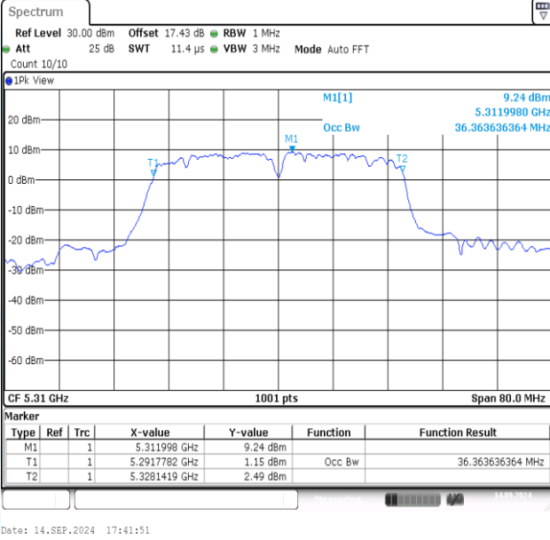
11N40MIMO-Ant1-5310
