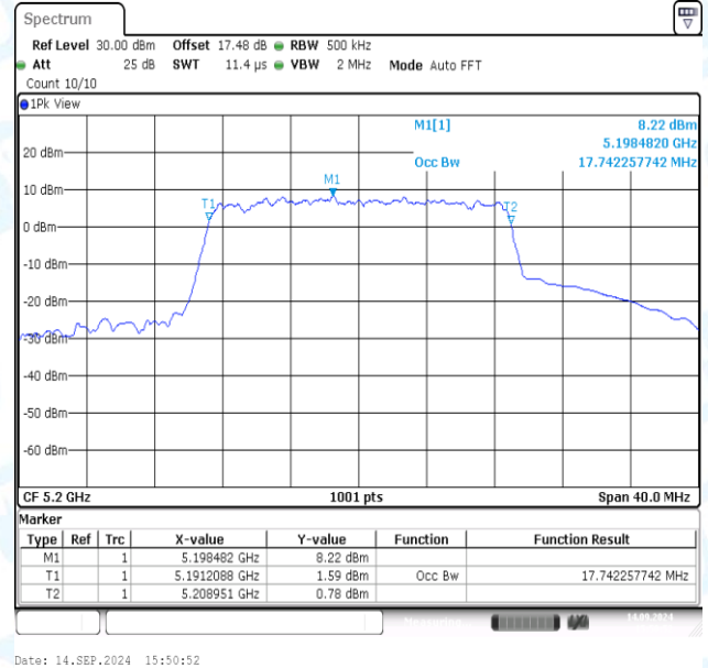
11N20MIMO-Ant2-5200
