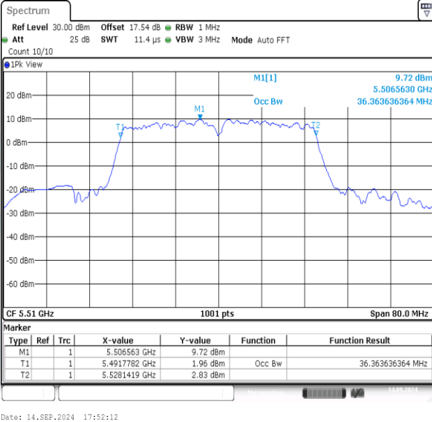
11N40MIMO-Ant1-5510
