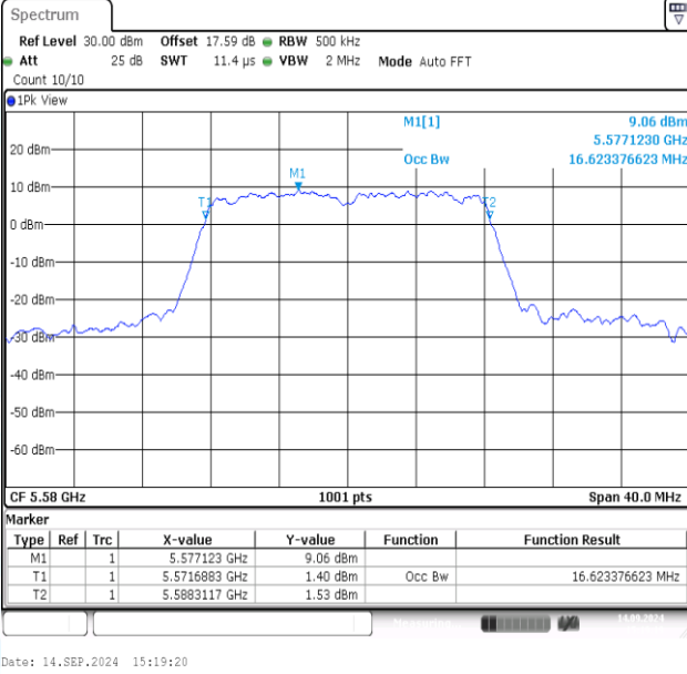
11A-Ant1-5580
