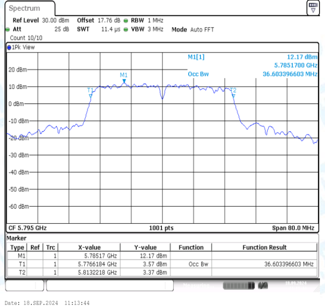
11N40MIMO-Ant2-5795
