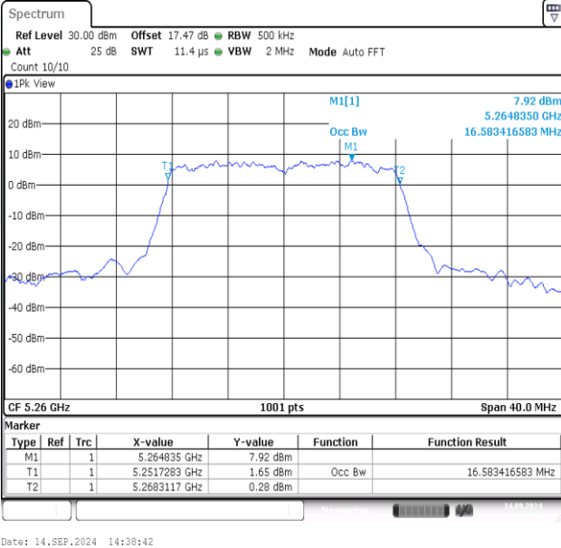
11A-Ant1-5260
