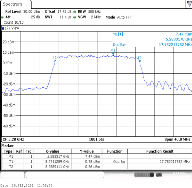
11AC20MIMO-Ant1-5280
