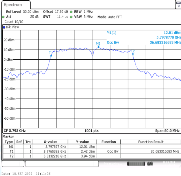
11N40MIMO-Ant1-5795
