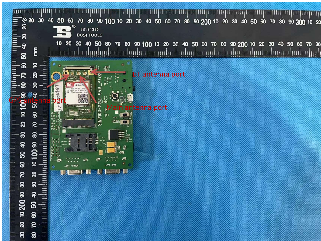
A7672SAminiPCIE
