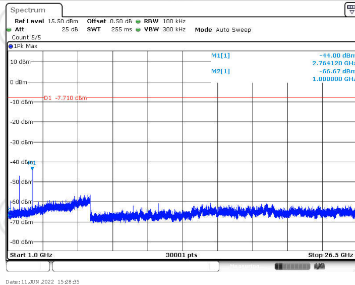
Ant1_921.4_1000~26500
