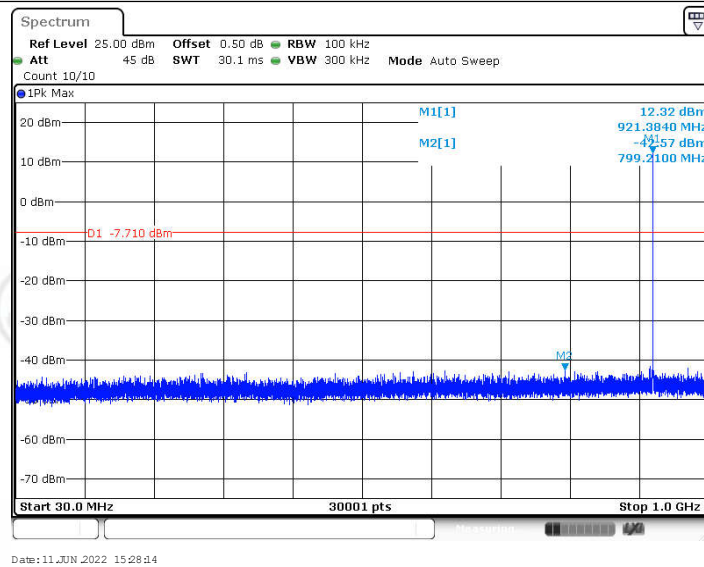
Ant1_921.4_30~1000
