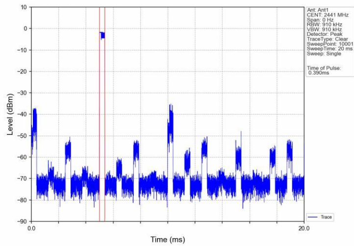
Pi/4DQPSK_2DH1_HOPP_Ant1_NTNV
