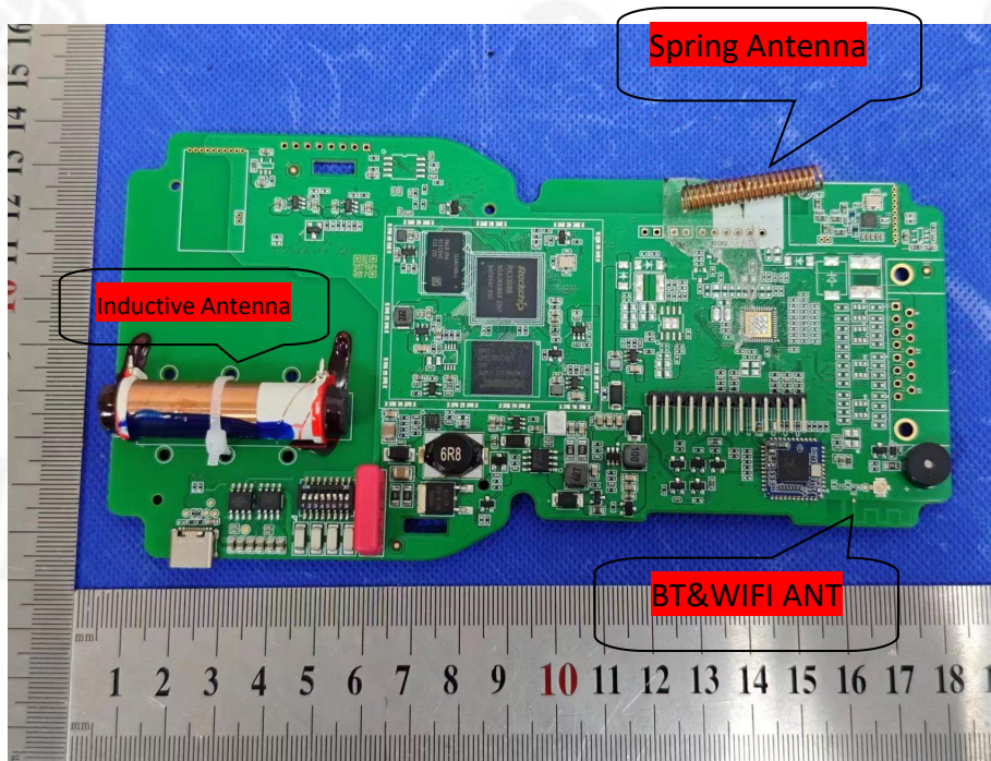
EUT Photo 4
