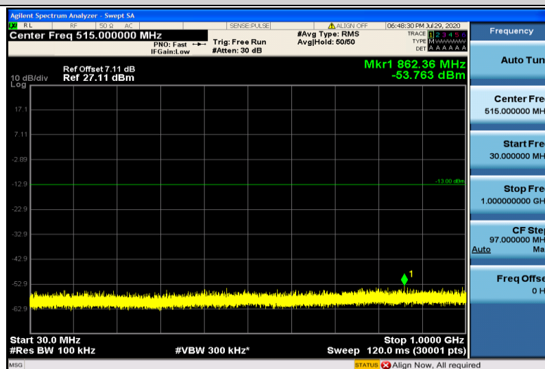
Band2-20MHz-16QAM-18700-1RB#0-30~1000MHz
