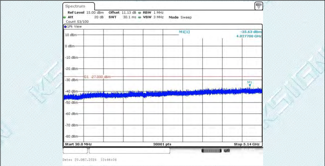
11N20ISO_Ant1_5320_30~5140
