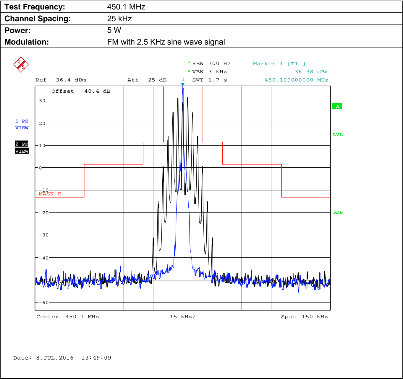
Plot 5.8.4.3.5. Emission Mask B, Low Power
