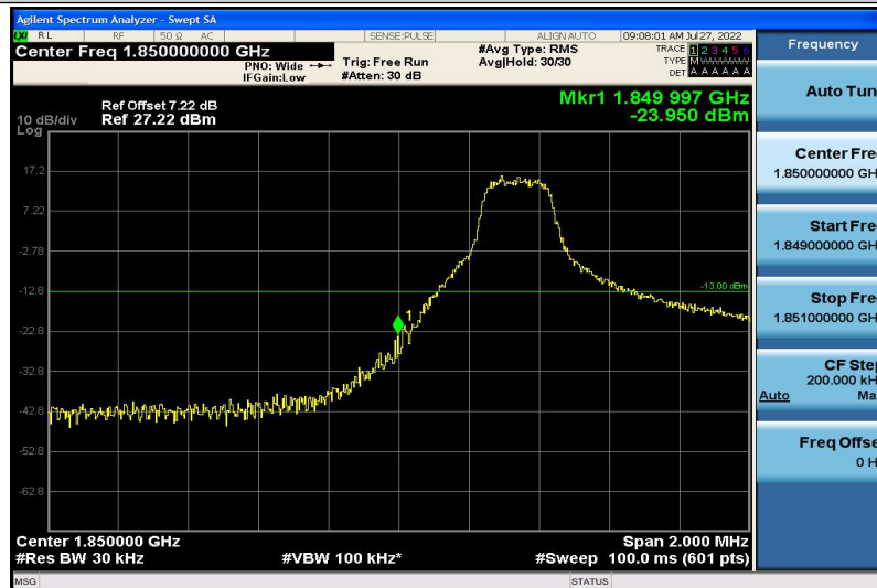
Band2-3MHz-QPSK-18615-1RB#0
