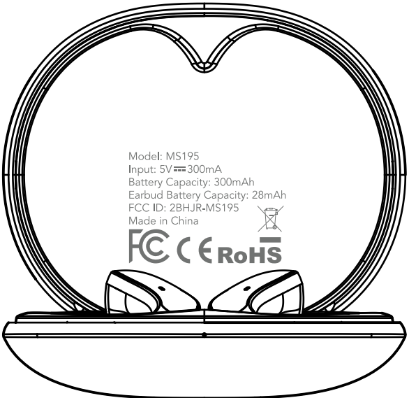
上盖内腔 丝印
