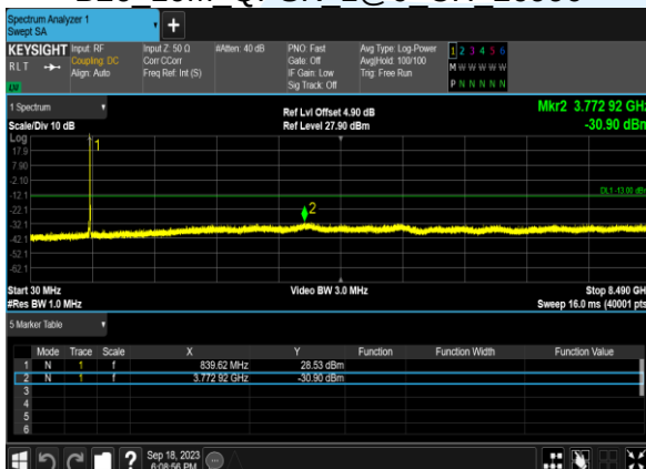
B26 10M QPSK 1@0 CH 26990
