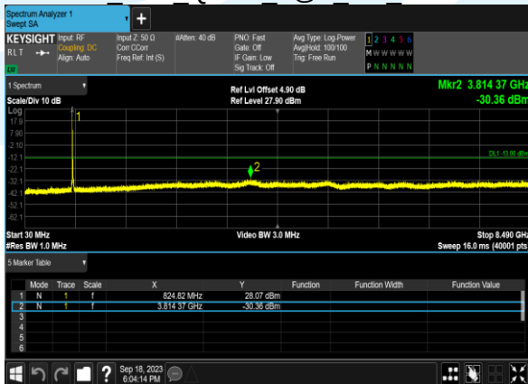
B26 15M QPSK 1@0 CH 26915
