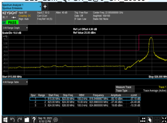
B26 15M QPSK 1@0 CH 26865
