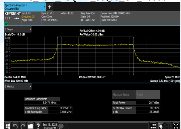
B26_10M 16QAM 50@0 CH 26990
