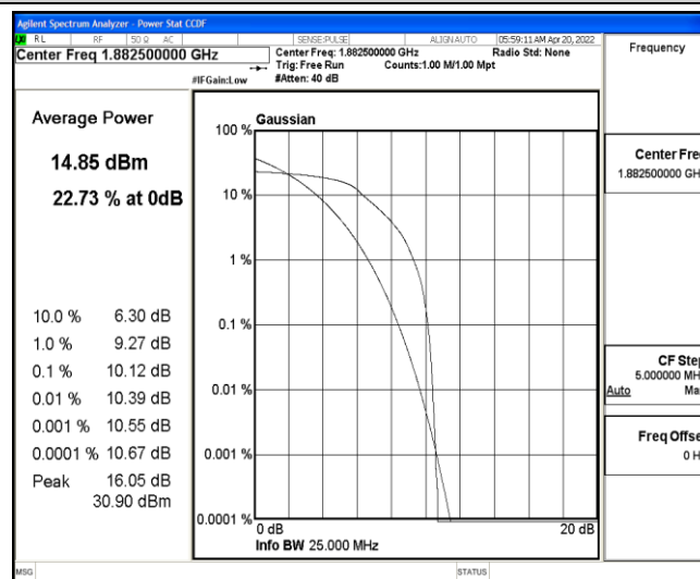
Band25-10MHz-QPSK-26365-6-0-Low-10.12-&lt;=13-PASS
