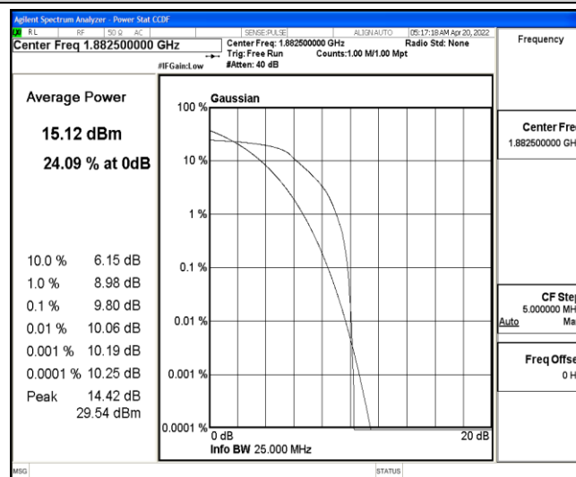
Band25-5MHz-QPSK-26365-6-0-Low-9.80-&lt;=13-PASS
