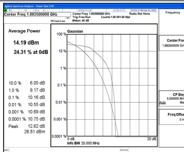
Band25-3MHz-QPSK-26365-6-0-Low-10.16-&lt;=13-PASS
