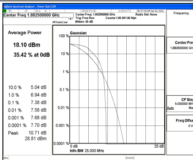
Band25-20MHz-QPSK-26365-6-0-Low-7.38-&lt;=13-PASS
