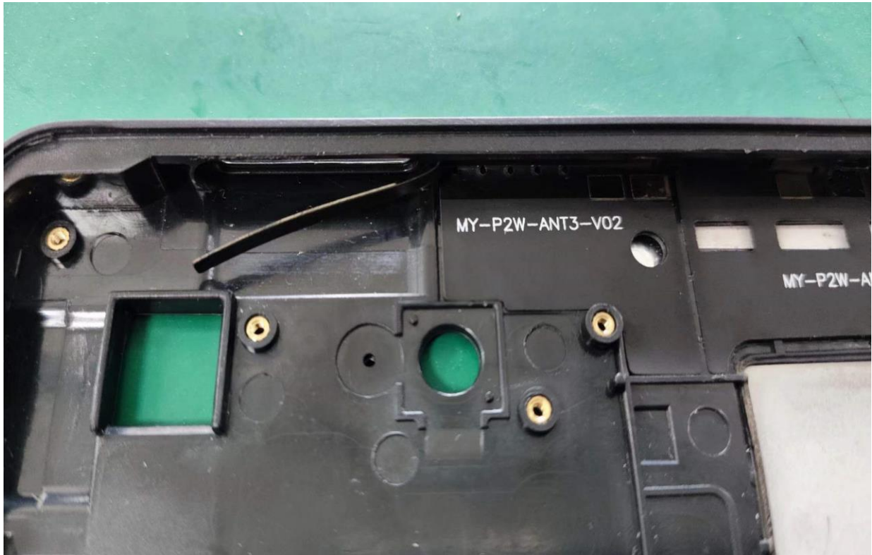
4G Div Ant MHB(PCS1900 W1/2/4 LTE B2/4/7/38/40/41/66)/2.4GWIFI/5G WIFI
