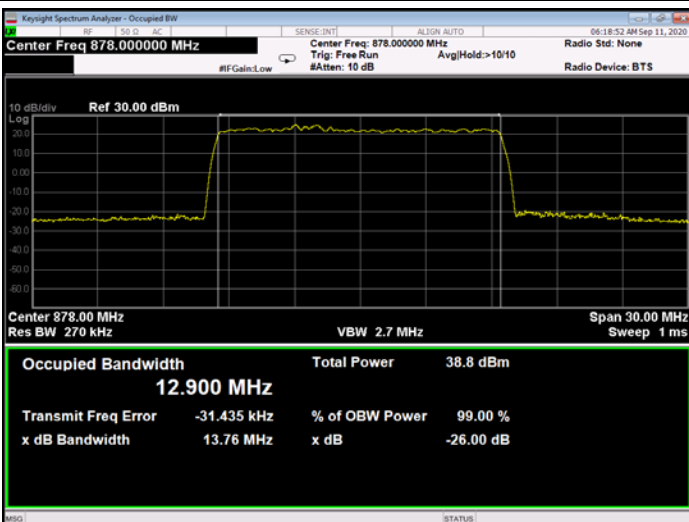
Figure 406: 64QAM 15MHz B.W.; 878.0MHz, 60kHz - Output
