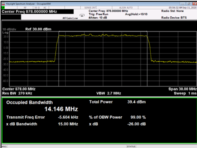
Figure 404: 64QAM 15MHz B.W.; 878.0MHz, 15kHz - Output
