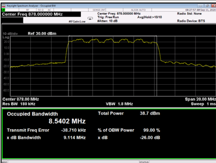
Figure 354: 16QAM 10MHz B.W.; 878.0MHz, 30kHz- Output
