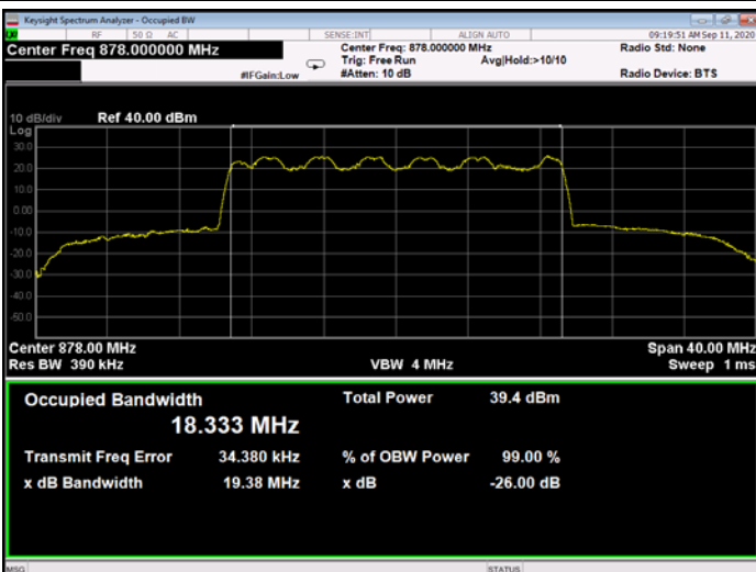
Figure 372: 16QAM 20MHz B.W.; 878.0MHz, 30kHz - Output
