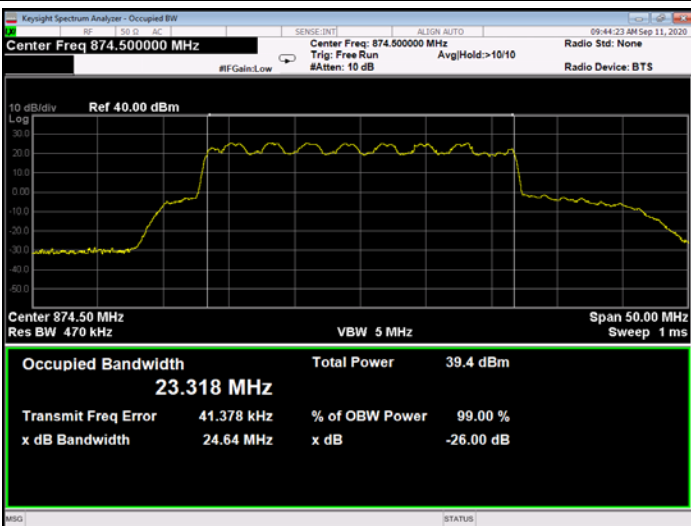
Figure 378: 16QAM 25MHz B.W.; 874.5MHz, 30kHz - Output
