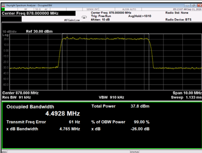
Figure 388: 64QAM 5MHz B.W.; 878.0MHz, 15kHz - Output
