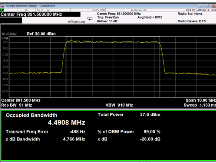
Figure 390: 64QAM 5MHz B.W.; 891.5MHz, 15kHz - Output
