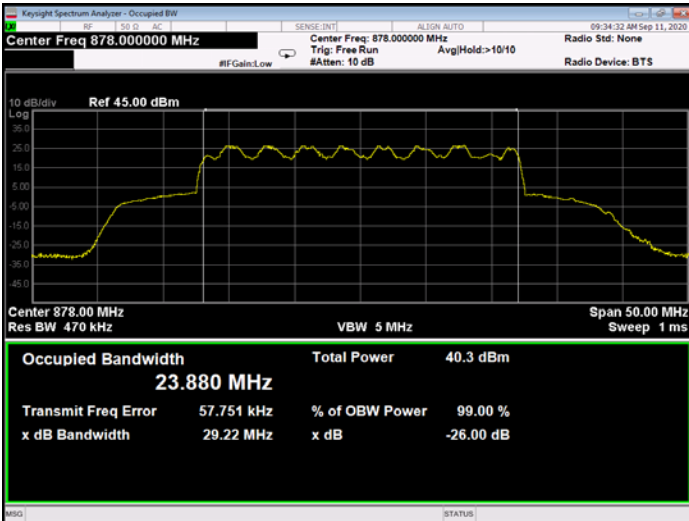
Figure 380: 16QAM 25MHz B.W.; 878.0MHz, 15kHz - Output
