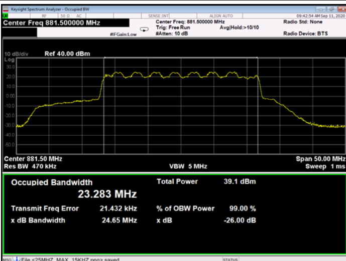
Figure 384: 16QAM 25MHz B.W.; 881.5MHz, 30kHz - Output
