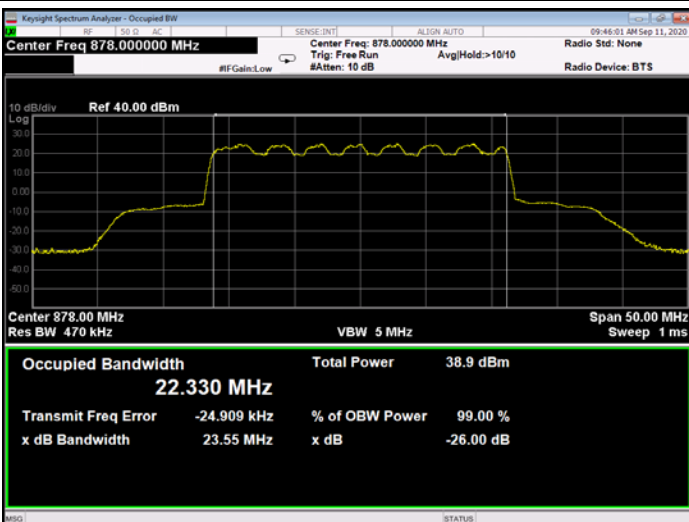
Figure 382: 16QAM 25MHz B.W.; 878.0MHz, 60kHz - Output
