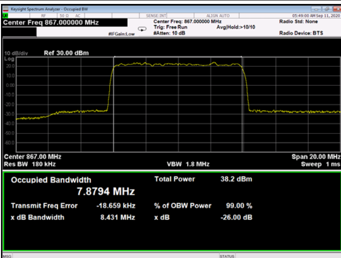
Figure 394: 64QAM 10MHz B.W.; 867.0MHz, 60kHz - Output
