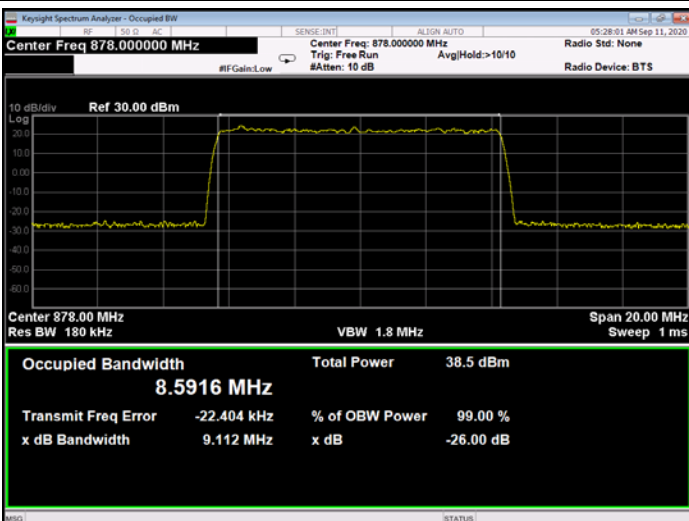
Figure 396: 64QAM 10MHz B.W.; 878.0MHz, 30kHz - Output
