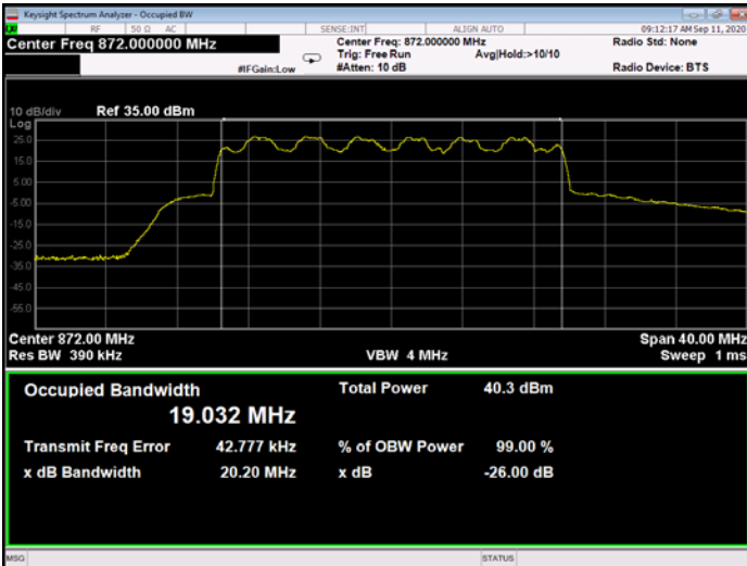
Figure 368: 16QAM 20MHz B.W.; 872.0MHz, 15kHz - Output
