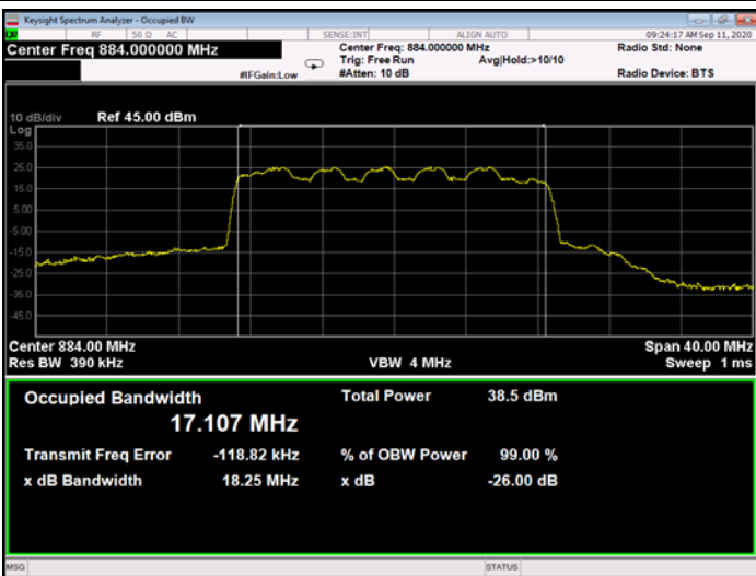
Figure 376: 16QAM 20MHz B.W.; 884.0MHz, 60kHz - Output
