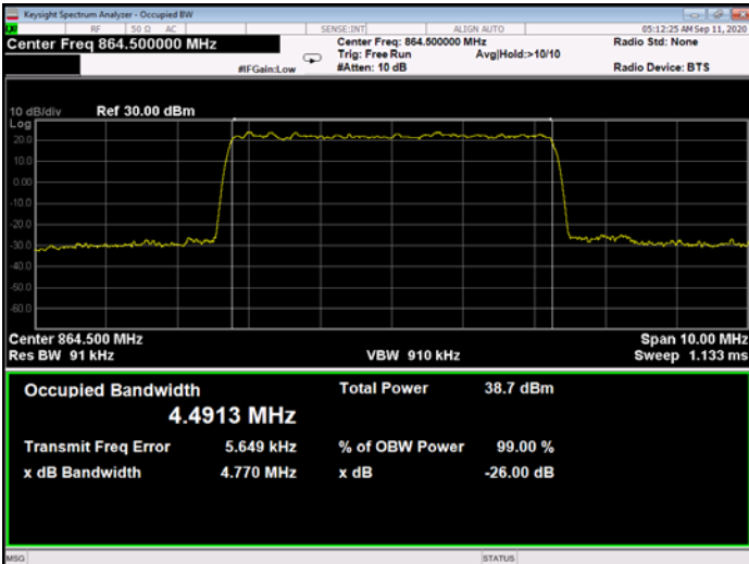
Figure 386: 64QAM 5MHz B.W.; 864.5MHz, 15kHz - Output
