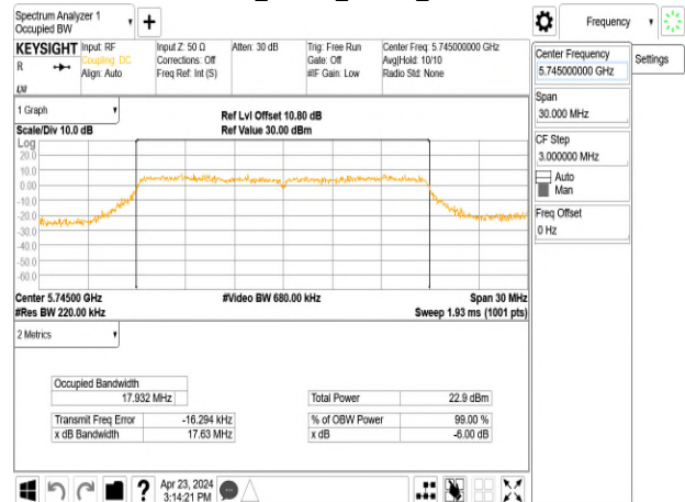
802.11n_20MHz_Chain0_5745MHz
